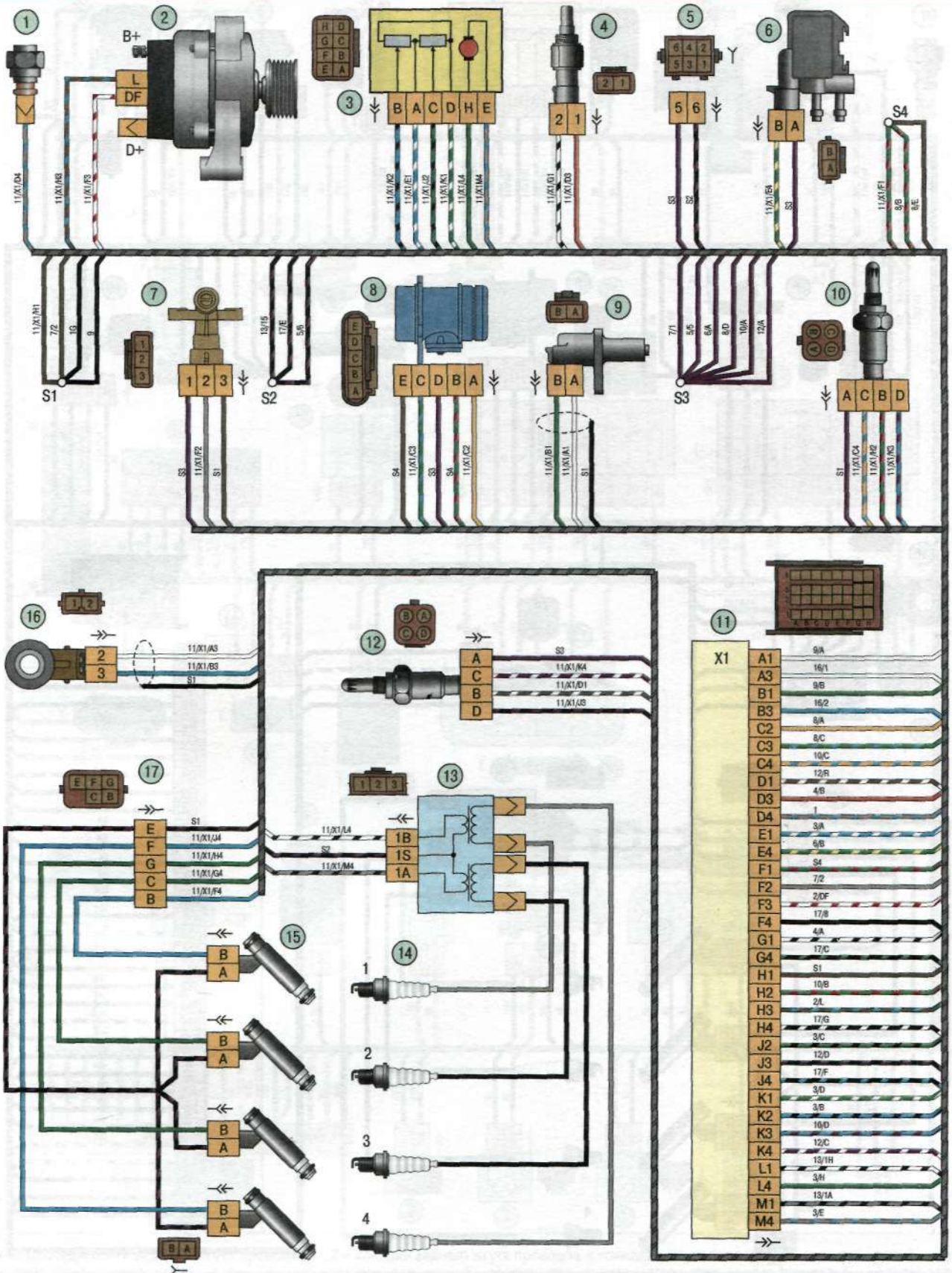
Схема 3. Соединения жгута проводов системы управления двигателями автомобиля без кондиционера: 1 - датчик сигнализатора аварийного падения давления масла; 2 - генератор; 3 - дроссельный узел; 4 - датчик температуры охлаждающей жидкости; 5 - колодка жгута проводов системы зажигания к колодке жгута проводов панели приборов; 6 - клапан продувки адсорбера; 7 - датчик скорости; 8 - датчик массового расхода воздуха; 9 - датчик положения коленчатого вала; 10 - управляющий датчик концентрации кислорода; 11 - электронный блок управления двигателем (контроллер); 12 - диагностический датчик концентрации кислорода; 13 - модуль зажигания; 14 - свеча зажигания; 15 - топливная форсунка; 16 - датчик детонации; 17 - колодка жгута проводов форсунок
