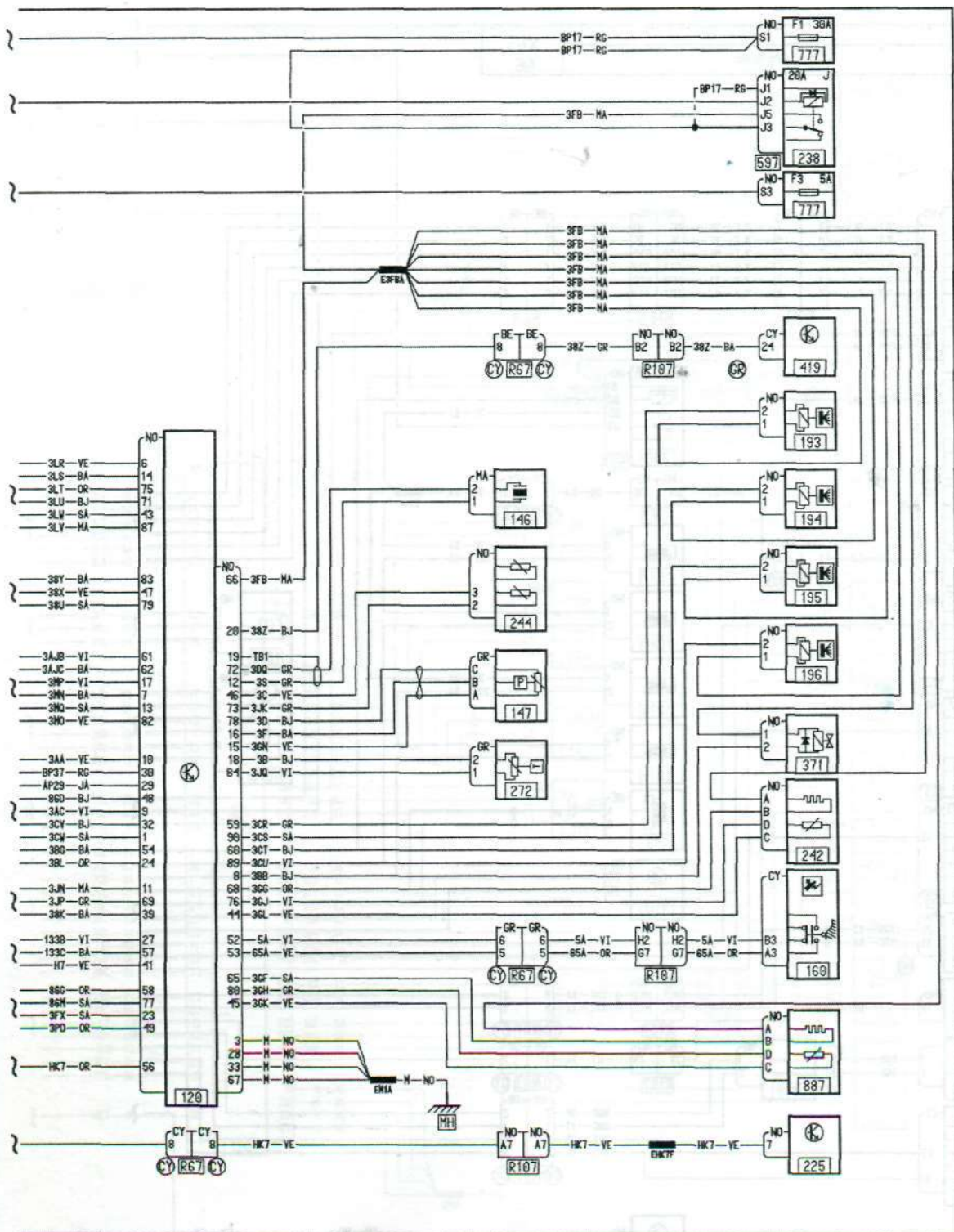
Система управления двигателем К4М 744 (2 из 2)
