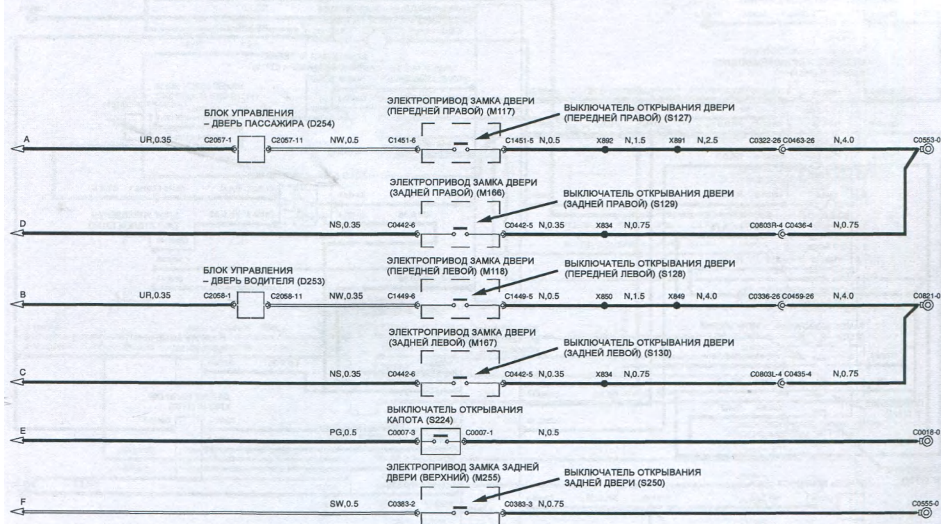
Схема 3-2. ПРОТИВОУГОННАЯ СИСТЕМА.
