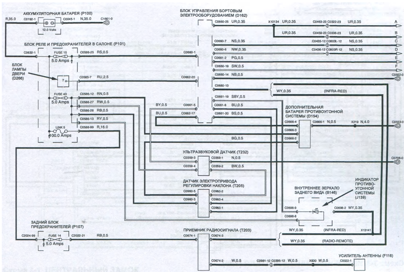
Схема 3-1. ПРОТИВОУГОННАЯ СИСТЕМА.
