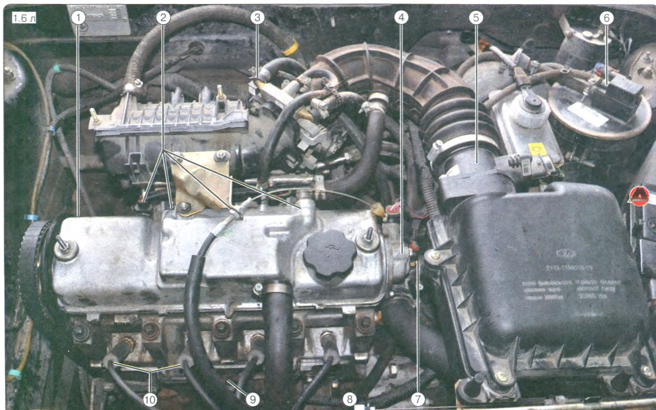
1. Датчик положения коленчатого вала, 2. Топливные форсунки, 3. Датчик положения дроссельной заслонки, 4. Датчик положения распределительного вала, 5. Датчик массового расхода воздуха, 6. Клапан продувки адсорбера, 7. Датчик температуры охлаждающей жидкости, 8. Модуль зажигания, 9. Датчик детонации, 10. Свечи зажигания
