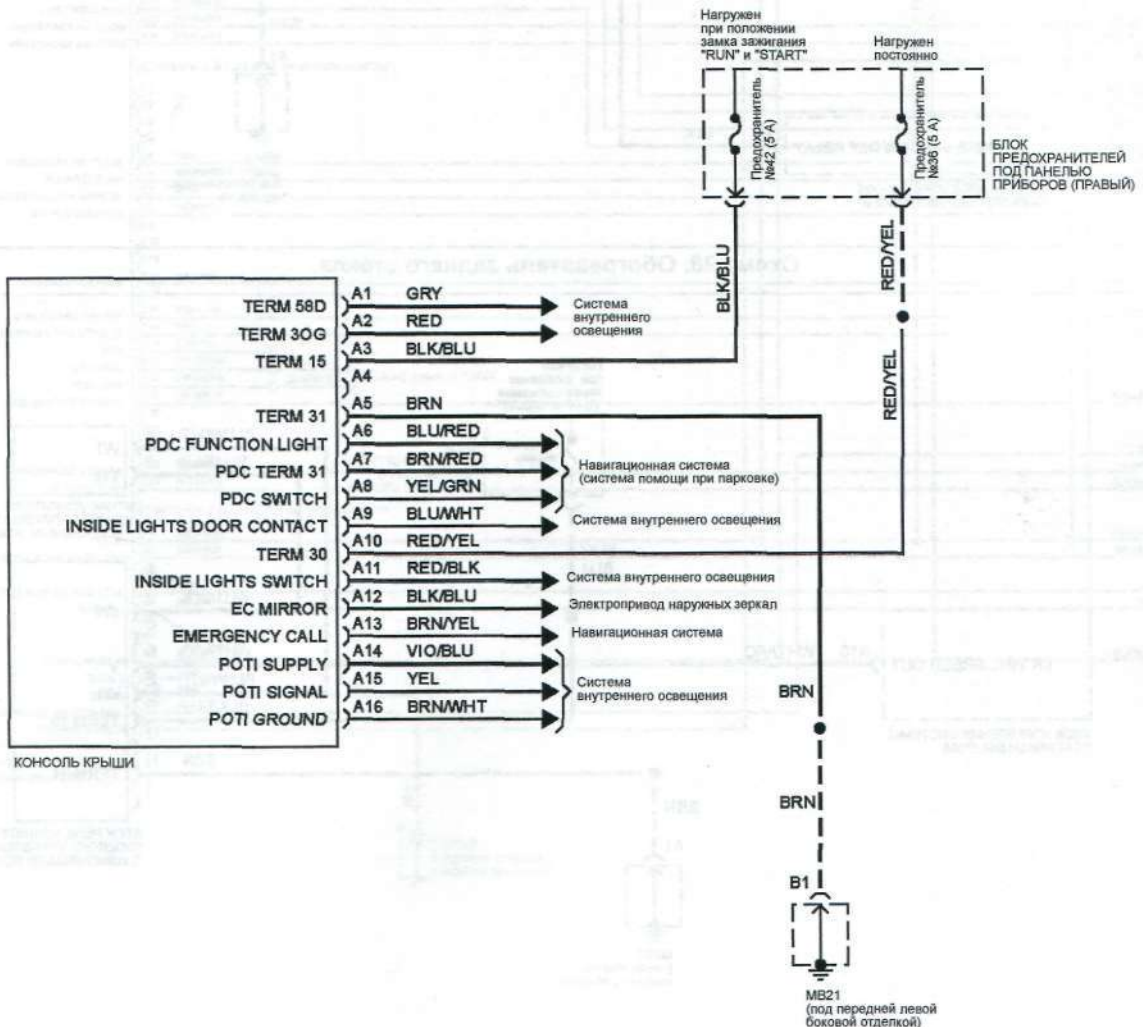
Схема 37. Консоль крыши.
