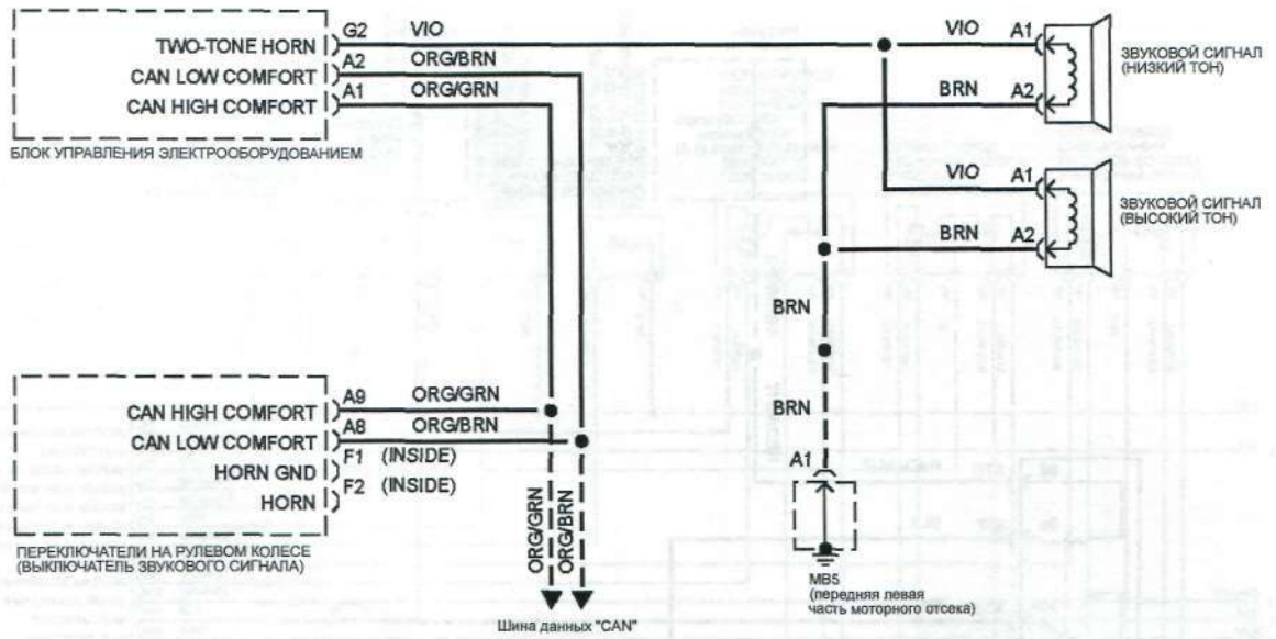
Схема 36. Звуковой сигнал.
