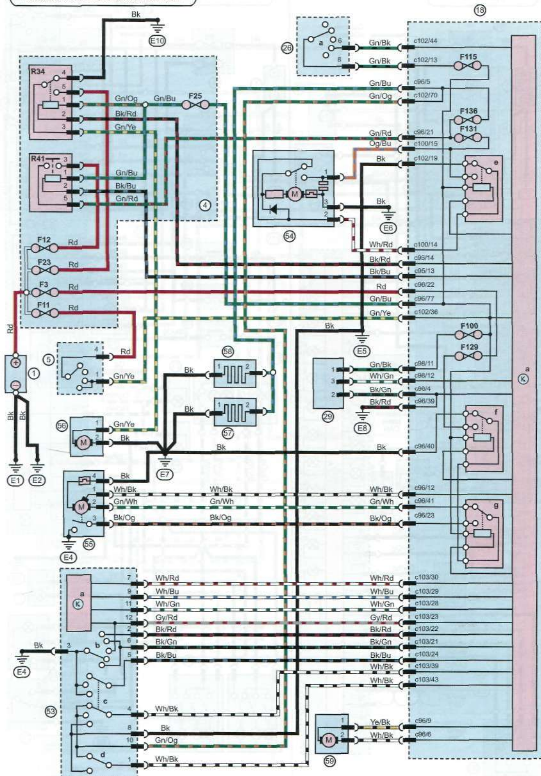
Типовая схема стеклоочистителей/омывателей
