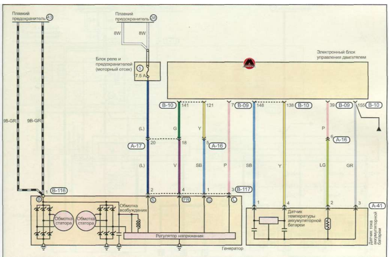
Система зарядки (модификация с двигателем 4N1) (часть 2).
