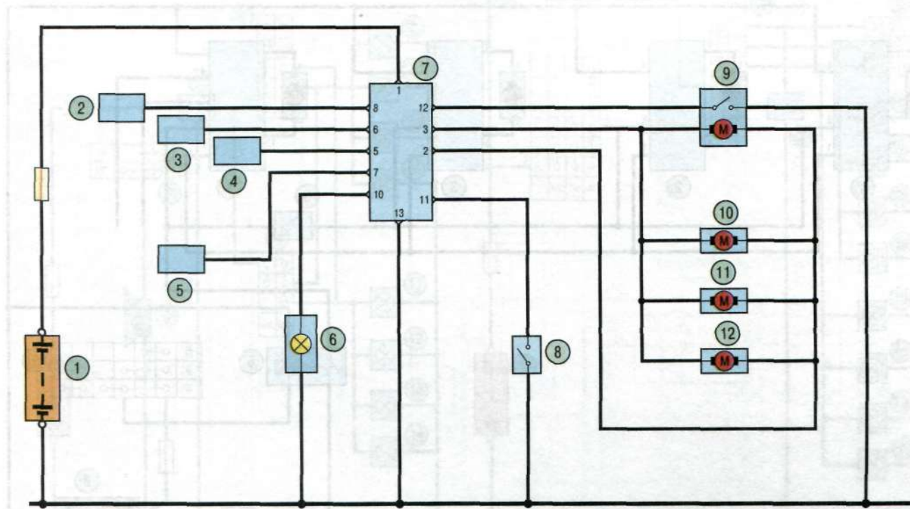
Схема 4. Центральный замок автомобиля Great Wall Safe: 1 – аккумуляторная батарея; 2 – к силовому проводу генератора; 3 – к левому фонарю бокового указателя поворота; 4 – к правому фонарю бокового указателя поворота; 5 – к концевому выключателю двери; 6 – блок фары автомобиля; 7 – блок управления центральным замком; 8 – клавиша блокировки и разблокировки замков дверей; 9 – привод замка левой передней двери; 10 – привод замка правой передней двери; 11 – привод замка левой задней двери; 12 – привод замка правой задней двери
