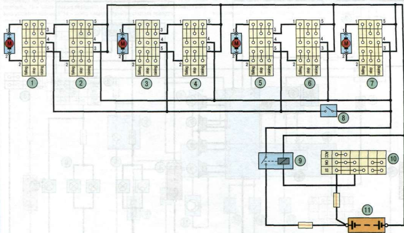
Схема 5. Стеклоподъемники автомобиля Great Wall Deer: 1 – дополнительная клавиша управления стеклоподъемником правой задней двери; 2 – основная клавиша управления стеклоподъемником правой задней двери; 3 – дополнительная клавиша управления стеклоподъемником левой задней двери; 4 – основная клавиша управления стеклоподъемником левой задней двери; 5 – дополнительная клавиша управления стеклоподъемником правой передней двери; 6 – основная клавиша управления стеклоподъемником правой передней двери; 7 – клавиша управления стеклоподъемником левой передней двери; 8 – кнопка блокировки управления стеклоподъемниками задних дверей; 9 – реле стеклоподъемников; 10 – выключатель (замок) зажигания; 11 – аккумуляторная батарея
