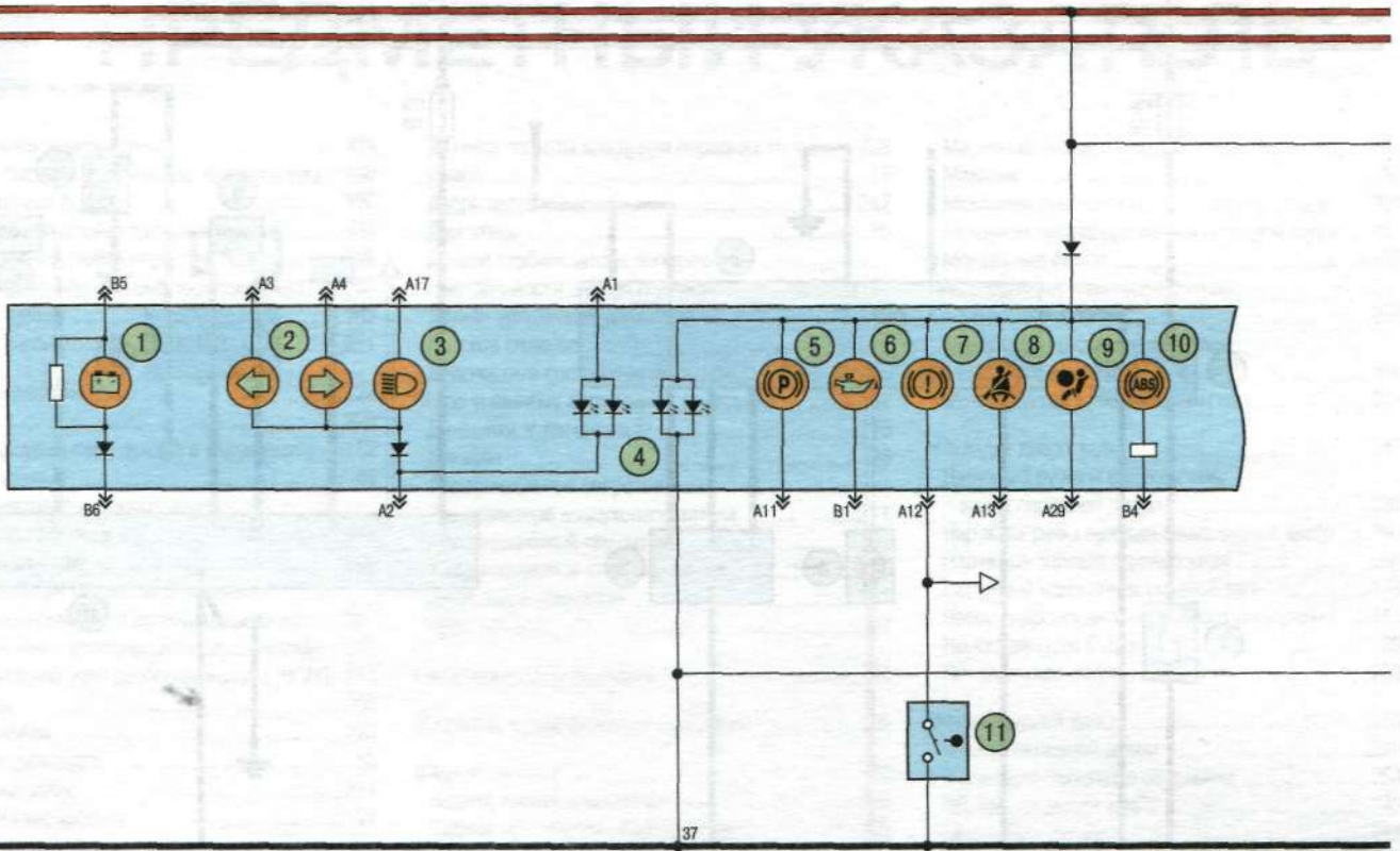
Схема 6а. Комбинация приборов: 1 – сигнализатор разряда аккумуляторной батареи; 2 – сигнализаторы указателей поворота; 3 – сигнализатор включения дальнего света фар; 4 – светодиоды подсветки; 5 – сигнализатор включения стояночного тормоза; 6 – сигнализатор аварийного давления масла; 7 – сигнализатор неисправности тормозной системы; 8 – сигнализатор непристегнутого ремня безопасности; 9 – сигнализатор неисправности системы подушек безопасности; 10 – сигнализатор антиблокировочной системы тормозов; 11 – датчик низкого уровня тормозной жидкости
