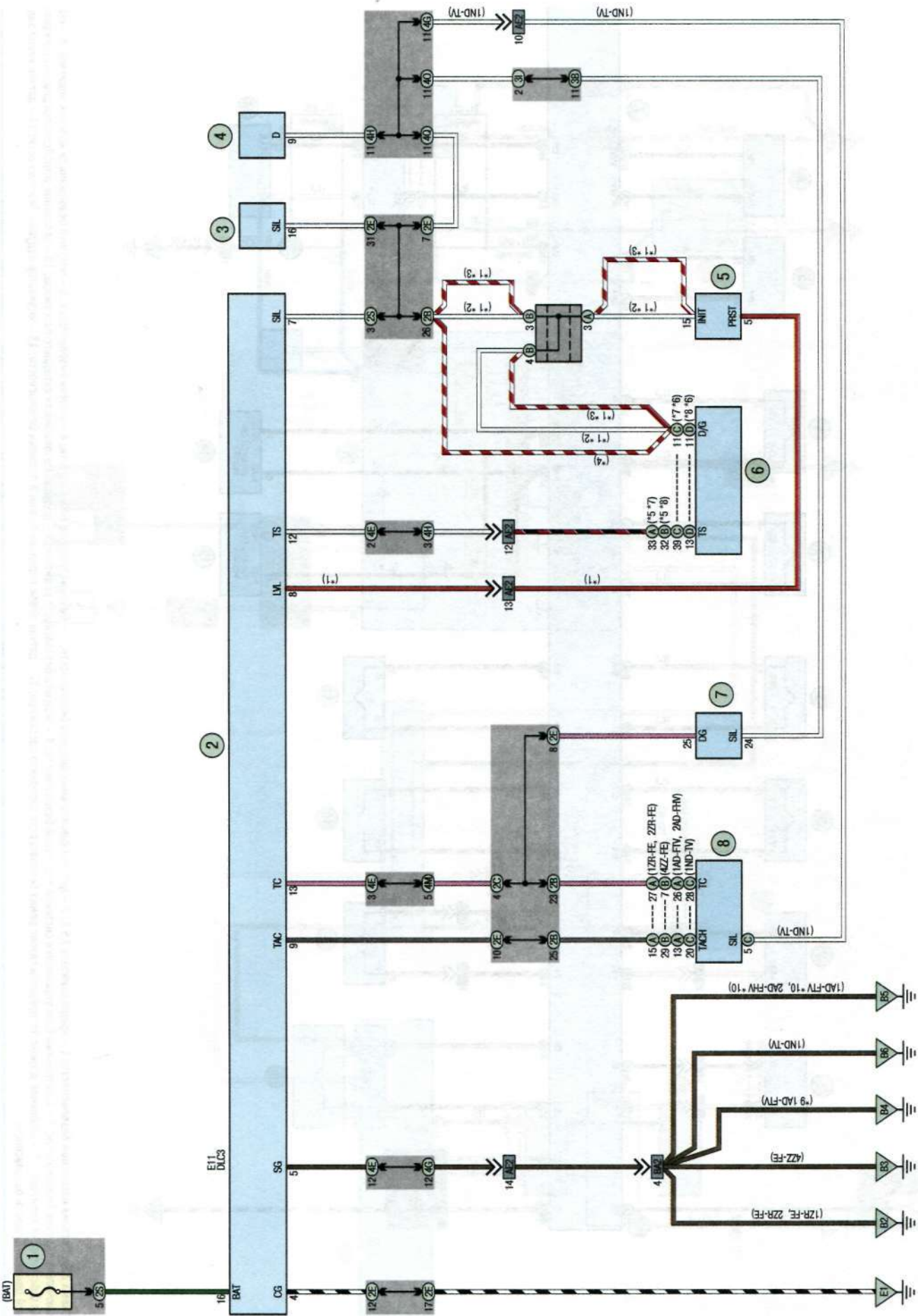
Схема 21. Диагностический разъем: 1 – предохранитель 7,5 А; 2 – датчик системы поддушек безопасности; 4 – иммобилайзер; 5 – блок управления автоматическим корректором света фар; 6 – блок управления ABS; 7 – блок управления роботизированной (автоматической) коробкой передач; 8 – ЭБУ двигателя
