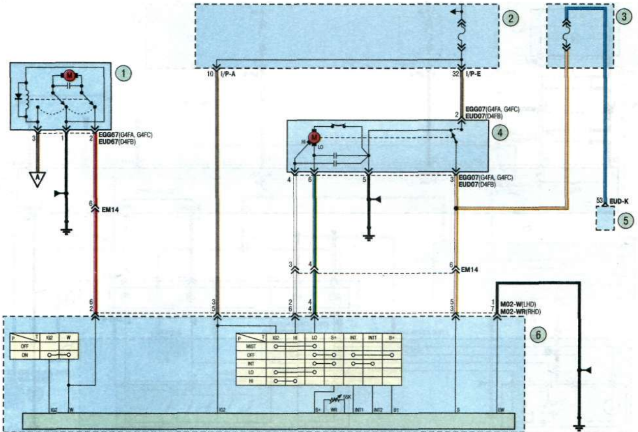
схема 20. Стеклоочистители и стеклоомыватель ветрового окна: 1 – электронасос омывателя; 2 – монтажный блок в салоне автомобиля; 3 – монтажный блок в моторном отсеке; 4 – моторредуктор переднего стеклоочистителя; 5 – электронный блок управления двигателем; 6 – переключатель стеклоочистителя и стеклоомывателя ветрового окна
