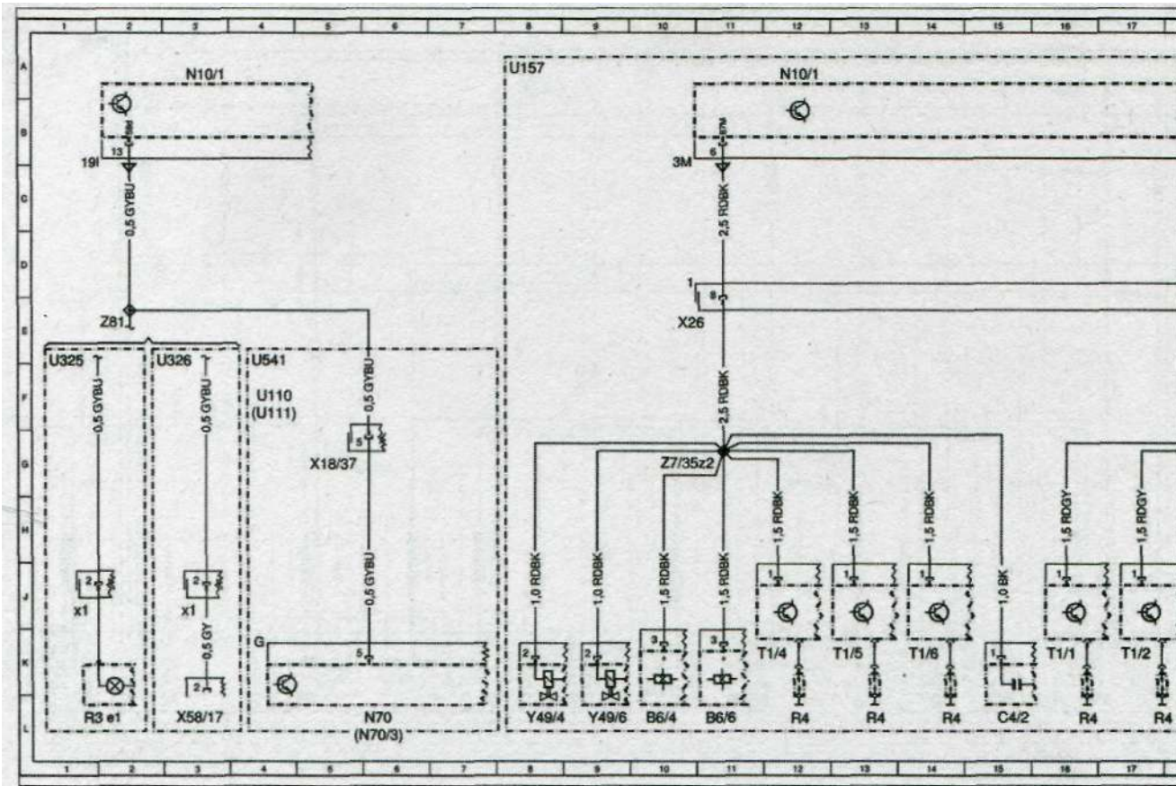
Электрическая схема блоков электрических соединений (Z) Z81, Z7/35 (M272 DE), Z7/36 (M272 DE), Z7/36z1 (M272 DE), Z7/38z1 (M272 DE), Z7/38z2 (M272 DE), Z7/39 (M272 DE), Z7/35z1 (M271 DE), Z7/35z2 (M271 DE), Z7/35z3 (M271 DE), Z7/36 (M271 DE), Z7/36z1 (M271 DE), Z7/36z2 (M271 DE), Z7/3, лист 3
