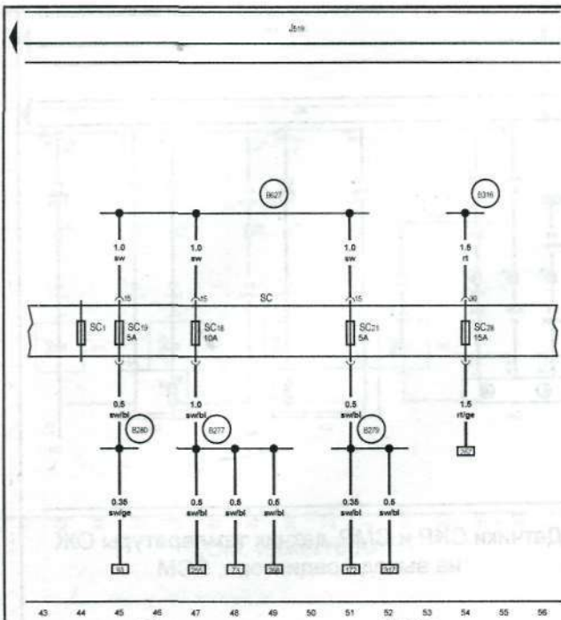
Блок предохранителей SC
