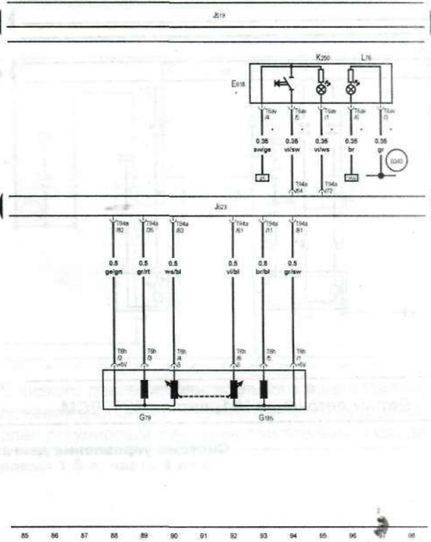
Выключатель противооткатной системы, датчик положения педали газа, ECM * специальное оборудование
