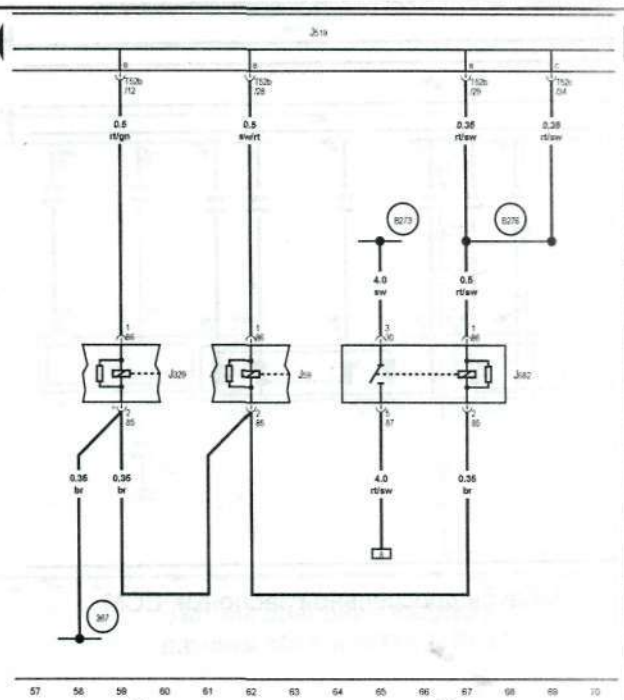
Реле разгрузки клеммы X, реле подачи питания клемм 15 и 50
