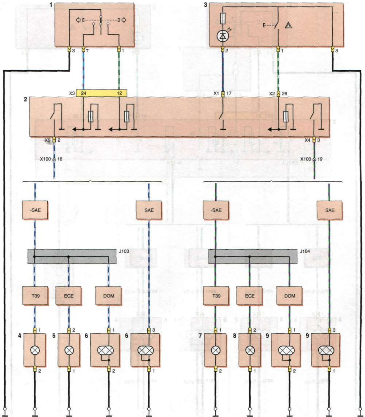
Схема включения передних указателей поворота и аварийной сигнализации: 1 – правый подрулевой переключатель; 2 – коммутационный блок; 3 – выключатель аварийной сигнализации; 4 – лампа левого бокового указателя поворота; 5 – лампа указателя поворота в левой блок-фаре; 6 – лампа указателя поворота/стояночного света в левой блок-фаре; 7 – лампа правого бокового указателя поворота; 8 – лампа указателя поворота в правой блок-фаре; 9 – лампа указателя поворота/стояночного света в правой блок-фаре
