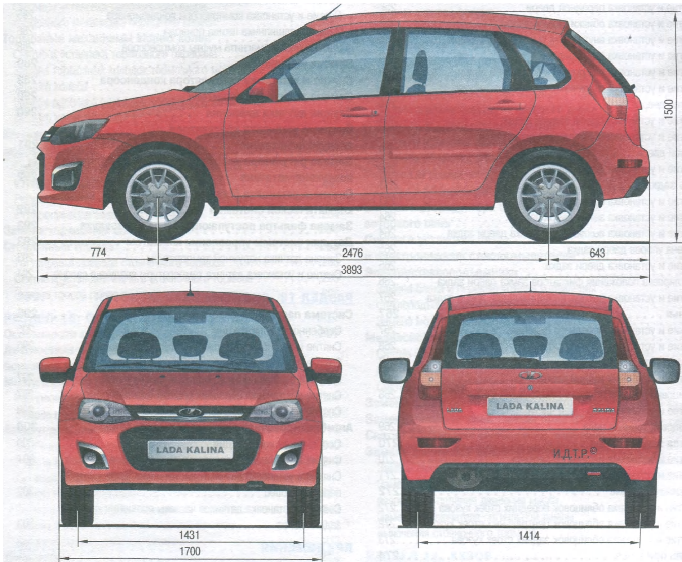
Рис. 1.1. Габаритные размеры автомобиля с кузовом хэтчбек
