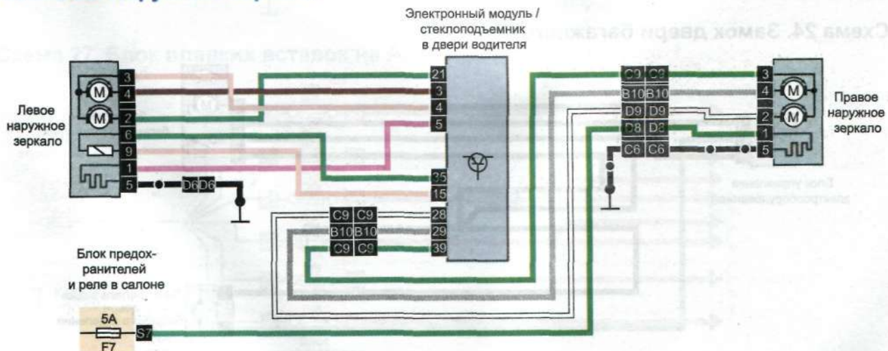
Схема 22. Наружные зеркала
