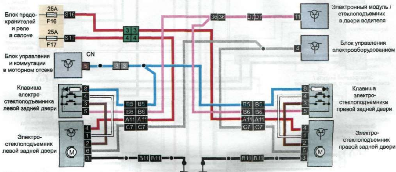
Схема 21. Электростеклоподъемники задних дверей
