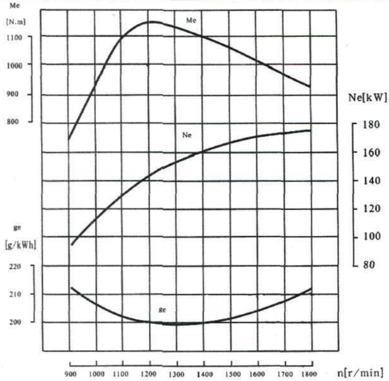
Двигатель WD 615.68GA-1
