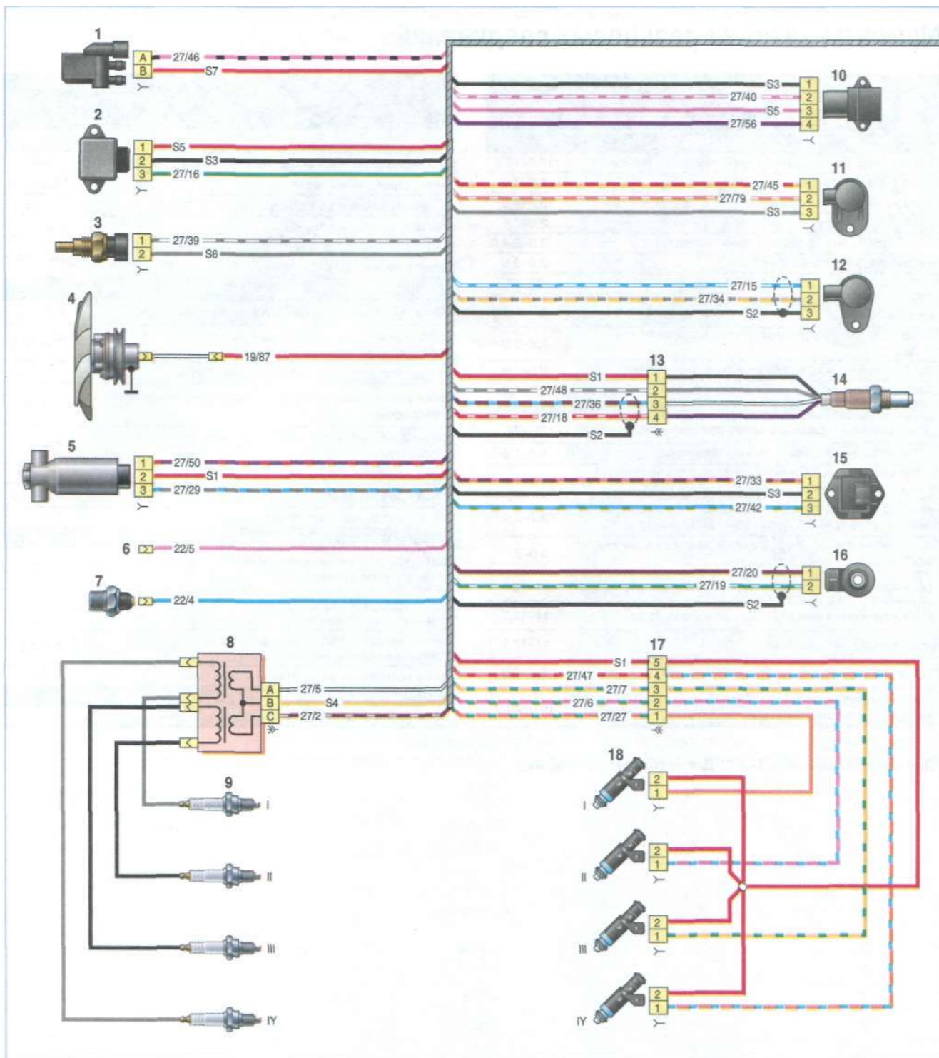
Схема соединений жгута проводов системы управления двигателем: 1 - клапан продувки адсорбера; 2 - датчик положения дроссельной заслонки; 3 - датчик температуры охлаждающей жидкости; 4 - муфта вентилятора; 5 - регулятор холостого хода; 6 - клемма D генератора; 7 - датчик сигнализатора аварийного давления масла; 8 - катушка зажигания; 9 - свечи зажигания; 10 - датчик абсолютного давления и температуры воздуха на впуске; 11 - датчик фаз; 12 - датчик положения коленчатого вала; J3 - колодка соединения со жгутом проводов управляющего датчика концентрации кислорода; 14 - управляющий датчик концентрации кислорода;
