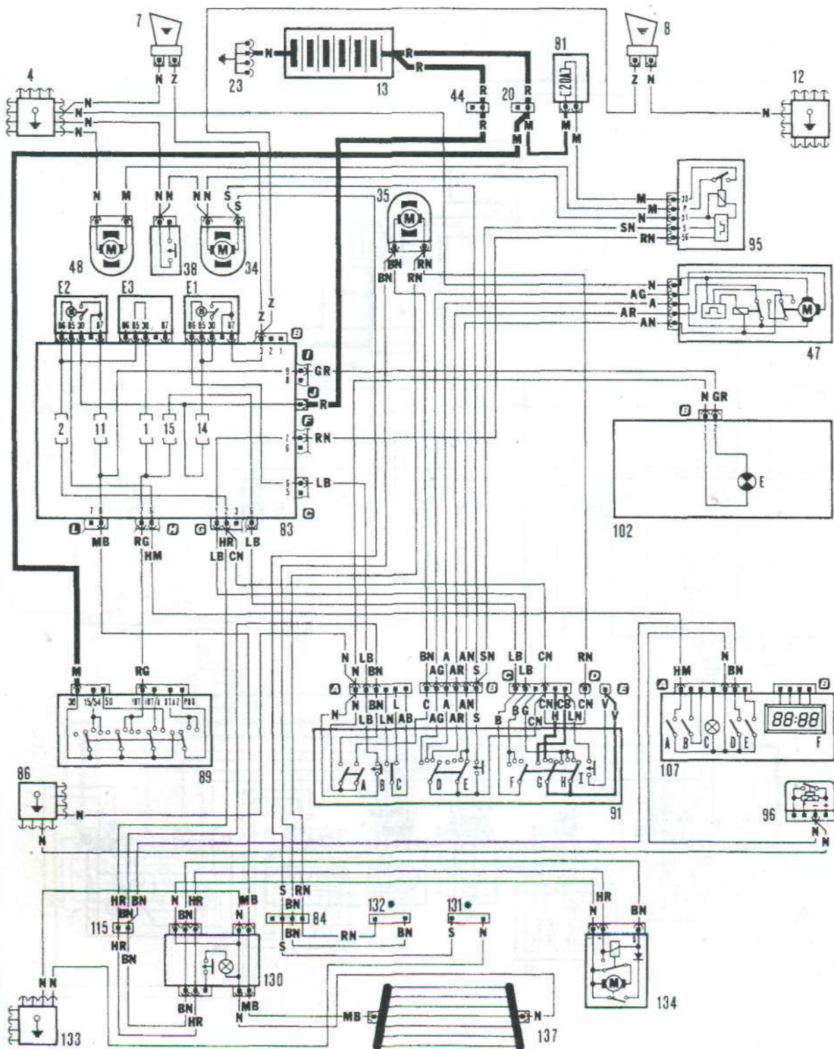
Схема 44: звуковые сигналы, обогреваемое заднее стекло, стеклоочиститель/омыватель переднего / заднего стекла и очиститель / омыватель фар (модель с двигателем 1372 см 3 TURBO ie) * расположение электрических насосов № 34 и 35, если подсоединен дополнительный омыватель фар
