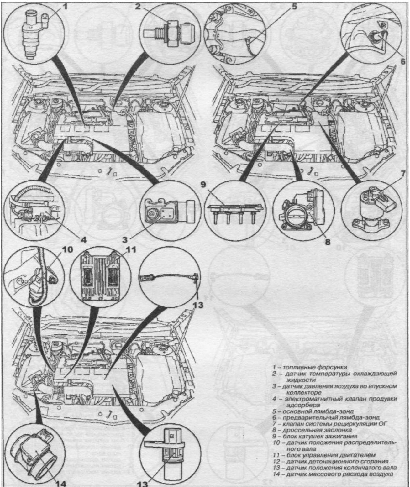
1. Компоненты системы впрыска Simtec 81 автомобиля с двигателем Z22YH
