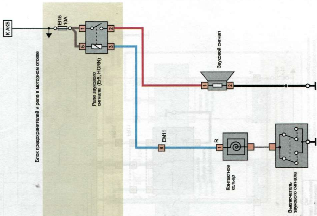
Схема 17. Звуковой сигнал
