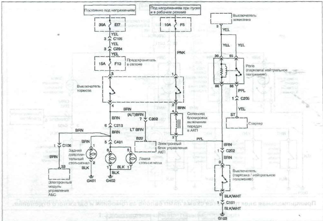
Принципиальная электрическая схема стоп-сигнала.
