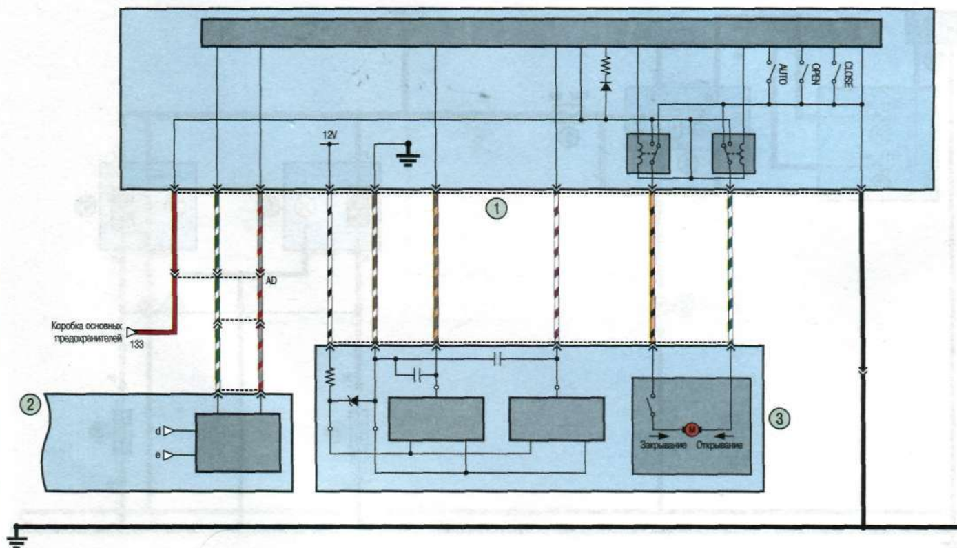
Схема 7г. Электростеклоподъемники: 1 – блок управления стеклоподъемниками; 2 – кнопка блокировки клавиш управления стеклоподъемниками правой передней и задних дверей; 3 – моторредуктор стеклоподъемника правой передней двери
