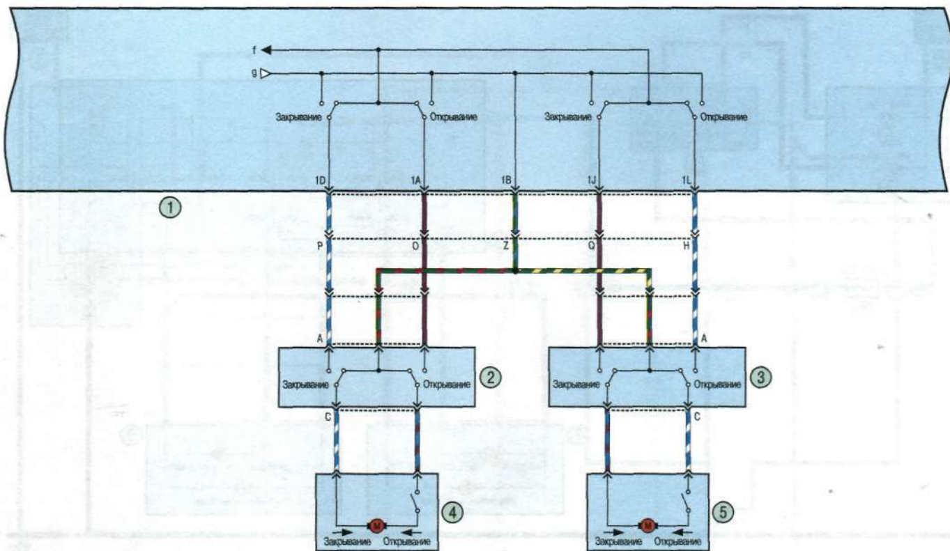
Схема 7в. Электростеклоподъемники: 1 – блок управления стеклоподъемниками; 2 – клавиша управления стеклоподъемником левой задней двери; 3 – клавиша управления стеклоподъемником правой задней двери; 4 – моторредуктор стеклоподъемника левой задней двери; 5 – моторредуктор стеклоподъемника правой задней двери
