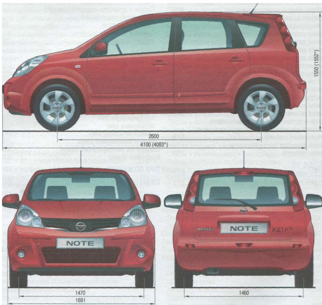
Рис. 1.1. Габаритные размеры автомобиля
