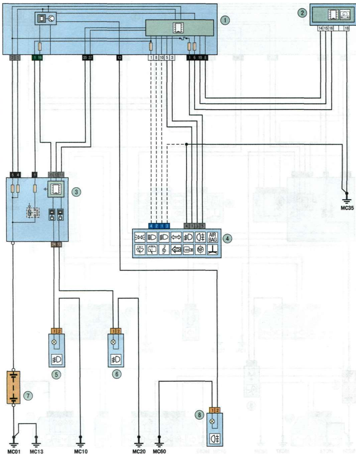
Схема 6. Противотуманные фары и фонари: 1 – блок управления электрооборудованием; 2 – панель приборов; 3 – монтажный блок в подкапотном пространстве; 4 – блок подрулевых переключателей; 5 – левая противотуманная фара; 6 – правая противотуманная фара; 7 – аккумуляторная батарея; 8 – задний противотуманный фонарь
