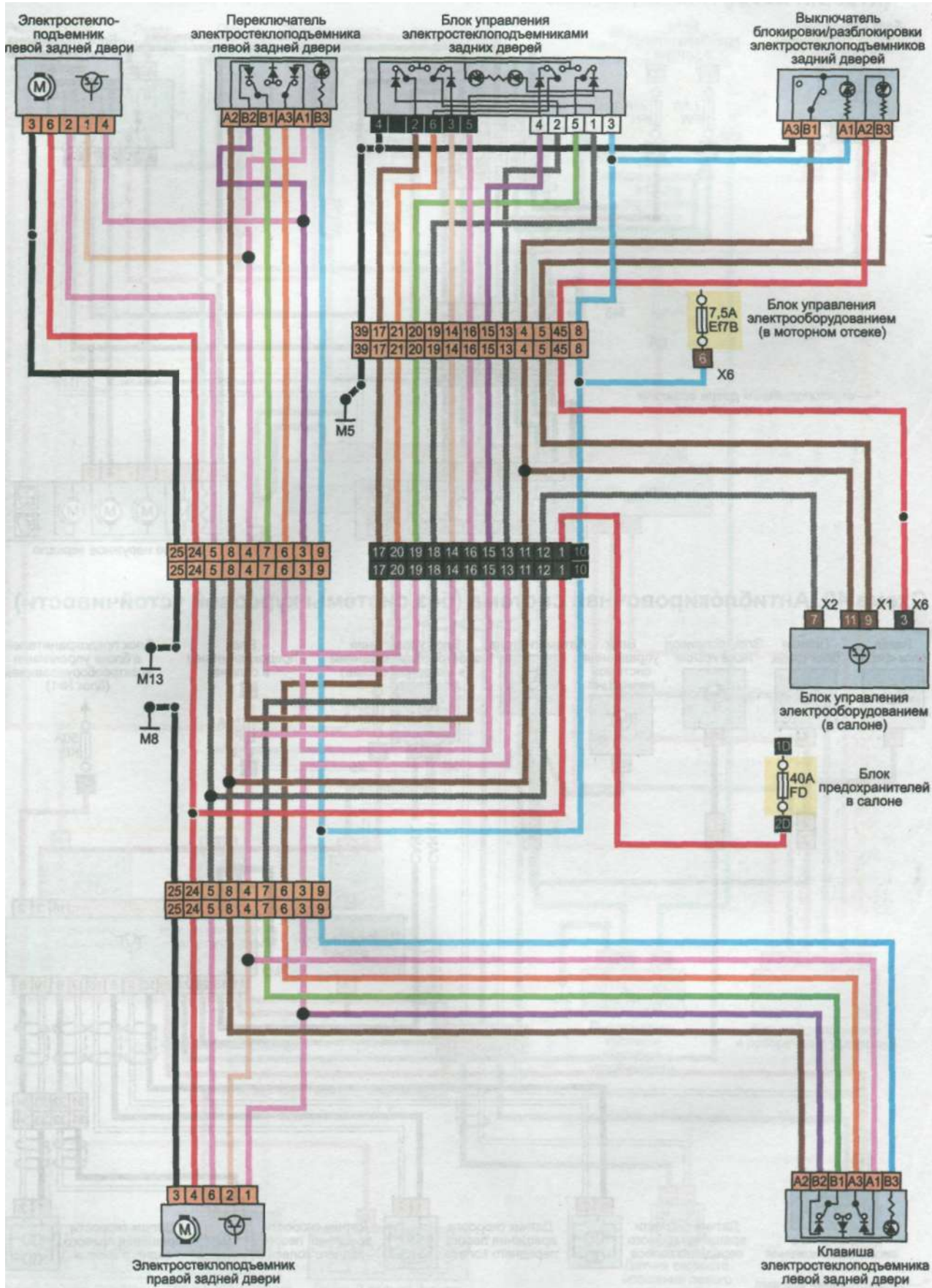
Схема 38. Электростеклоподъёмники задних дверей
