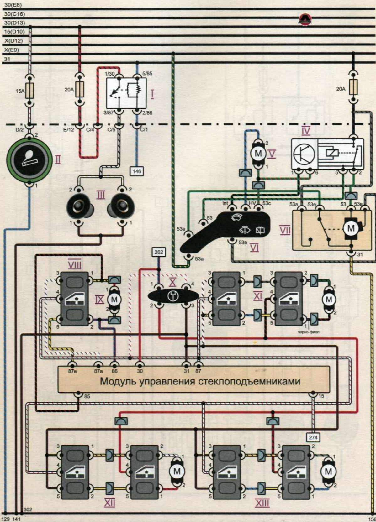
I. Реле очистителя ветрового стекла. II. Прикуриватель. III. Звуковой сигнал. IV. Реле очистителя ветрового стекла. V. Насос омывателя ветрового стекла. VI. Переключатель очистителя и омывателя ветрового стекла. VII. Очиститель ветрового стекла. VIII. Выключатель стеклоподъемника левой передней двери. IX. Электромотор стеклоподъемника. X. Выключатель блокировки задних стеклоподъемников. XI. Выключатель стеклоподъемника правой передней двери. XII. Выключатель стеклоподъемника левой задней двери. XIII. Выключатель стеклоподъемника правой задней двери.
