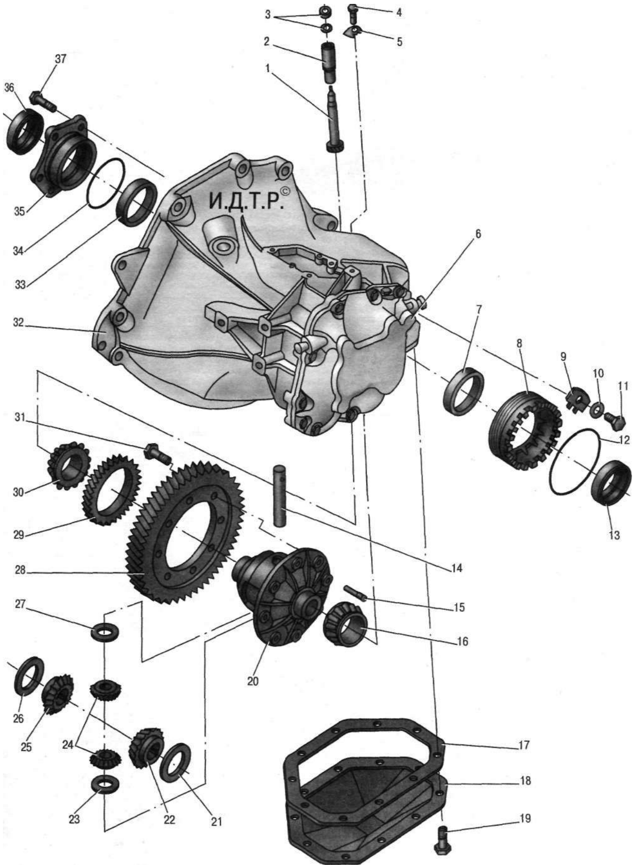
рис.6.6. Главная передача и дифференциал: 1 - вал-шестерня редуктора привода спидометра; 2 - корпус редуктора привода спидометра; 3, 12, 34 - уплотнительные кольца; 4 - стопорная пластина; 5 - стопорная пластина; 6 - задняя крышка коробки передач; 7, 33 - наружные кольца подшипников дифференциала; 8 - регулировочная гайка подшипников; 9 - пластина фиксатора; 10 - шайба; 11, 19, 31, 37 - болты; 12, 34 - уплотнительные кольца; 13, 36 - сальники; 14 - ось сателлитов дифференциала; 15 - фиксатор оси сателлитов; 16, 30 - конические роликовые подшипники дифференциала; 17 - прокладка; 18 - нижняя крышка коробки передач; 20 - корпус дифференциала; 21, 26 - упорные шайбы; 22, 25 - полусосевые шестерни; 23, 27 - упорные шайбы сателлитов; 24 - сателлиты; 28 - ведомая шестерня главной передачи; 29 - ведущая шестерня привода спидометра; 32 - картер коробки передач; 35 - правая крышка подшипников дифференциала
