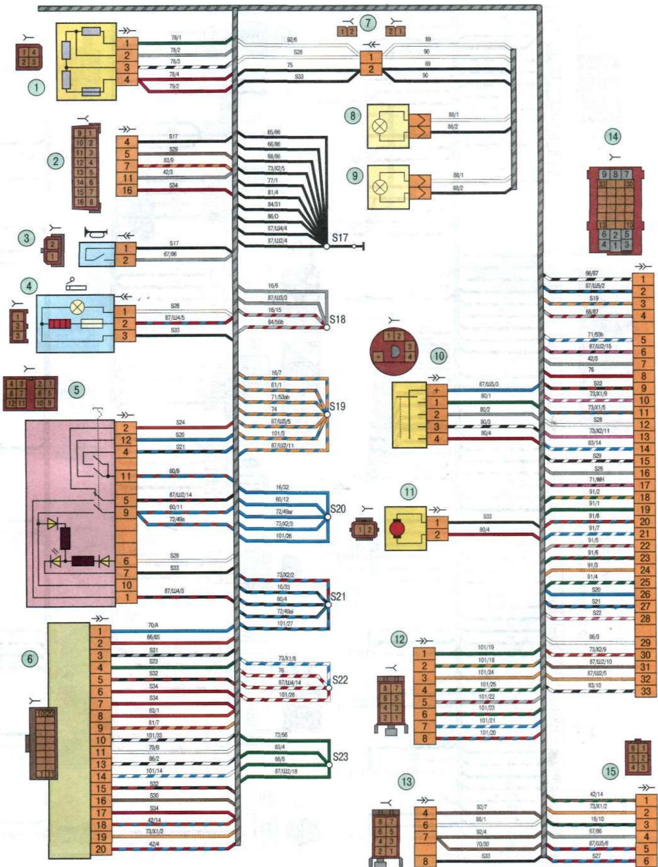
Приложение 10. Дополнительный жгут проводов панели приборов автомобиля выпуска с 2009 года: 1 – добавочное сопротивление; 2 – диагностический разъем; 3 – выключатель звукового сигнала; 4 – прикуриватель; 5 – выключатель аварийной сигнализации; 6 – блок управления противобуксировочной системой; 7 – колодка жгута подсветки панели управления климатом; 8, 9 – подсветка панели управления климатом; 10 – переключатель режимов работы воздуханогнетателя; 11 – электродвигатель воздуханогнетателя; 12, 13 – колодки жгута проводов к аудиосистеме; 14, 15 – колодка жгута панели приборов к заднему жгуту
