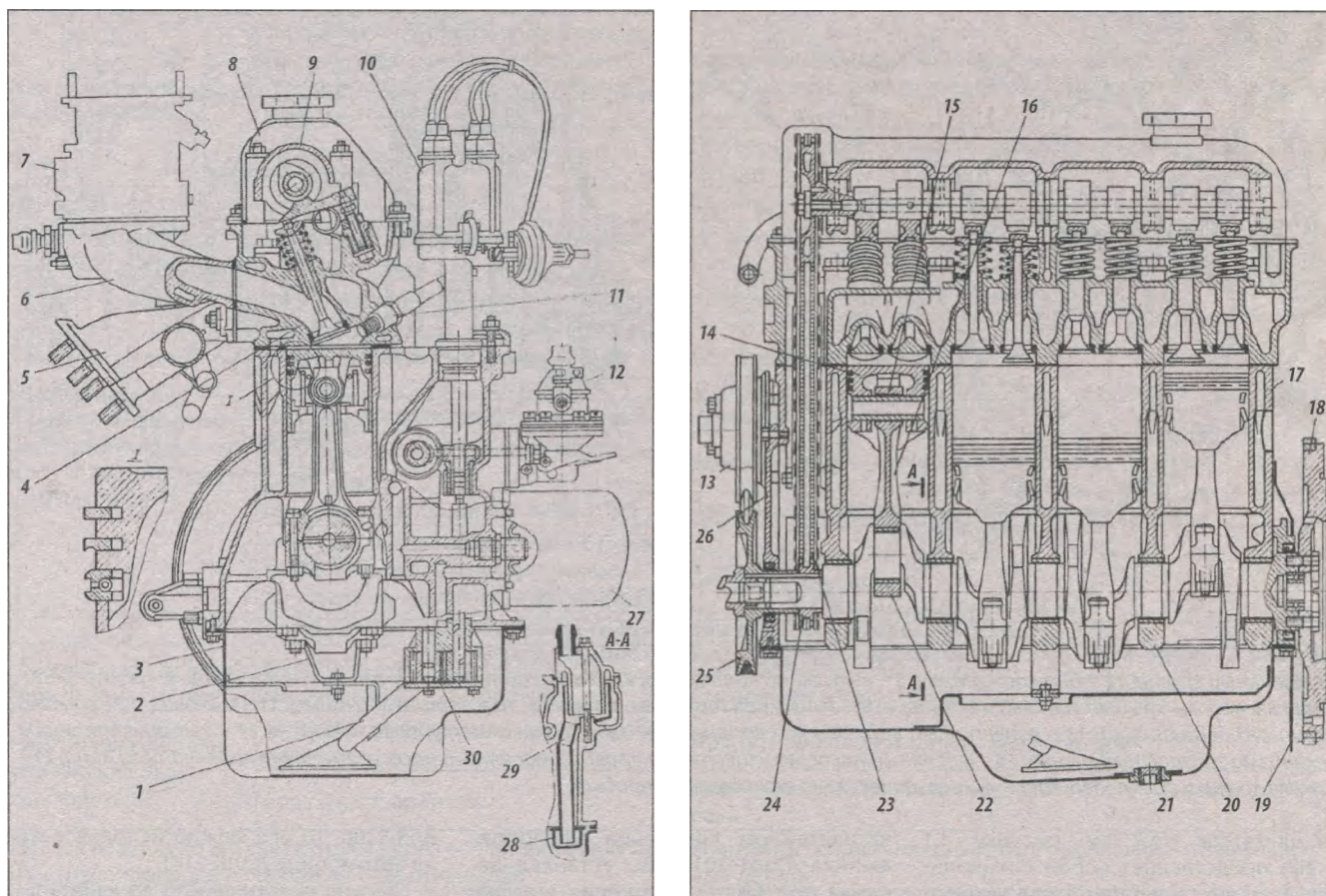
Рисунок 3.2. Поперечный и продольный разрезы двигателя ВАЗ:
