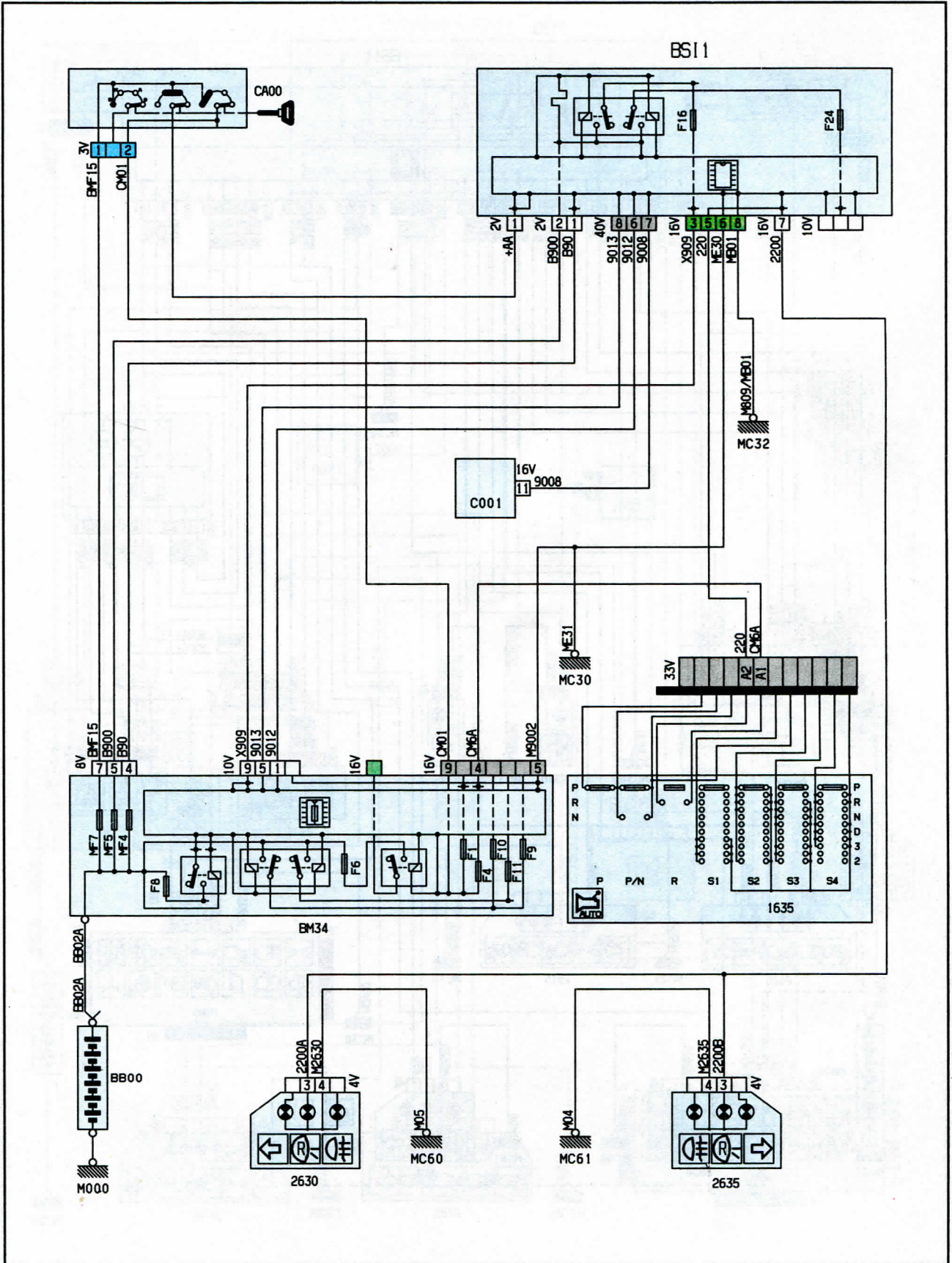
Схема 15. Фонари заднего хода. Автомобили с кузовом «универсал» и автоматической коробкой переключения передач
