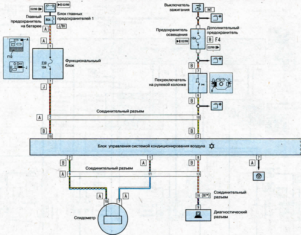
Схема 29. Система кондиционирования воздуха
