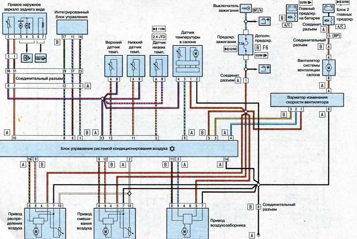
Схема 30. Система кондиционирования воздуха (окончание)
