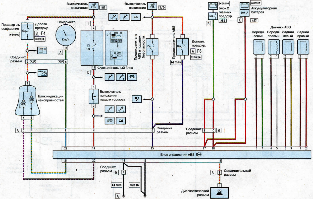
Схема 31. Антиблокировочная тормозная система (ABS)
