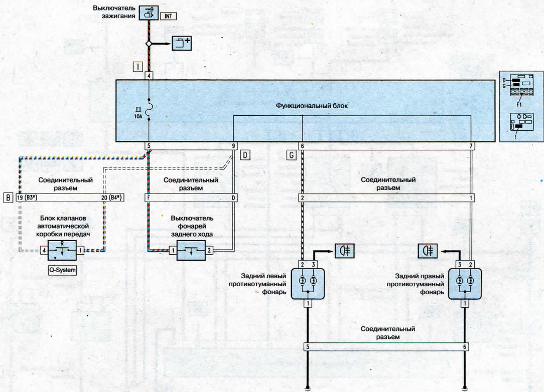
Схема 32. Фонари заднего хода
