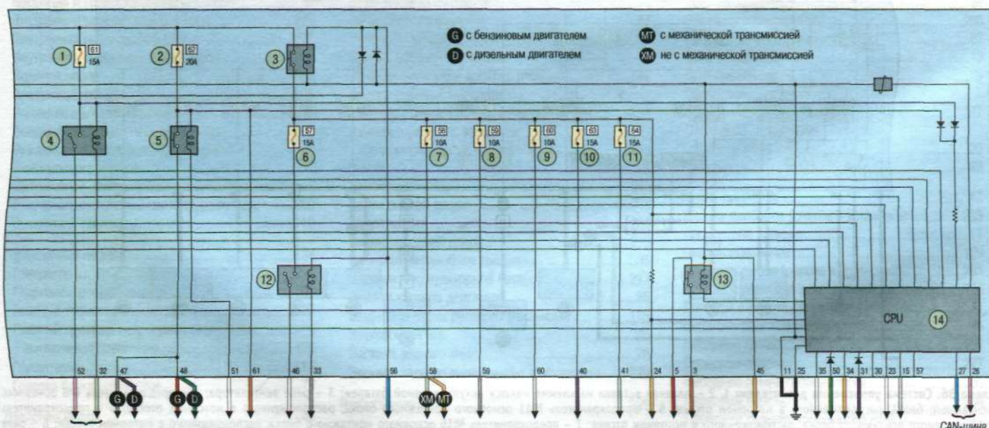
Схема 2б. Монтажные блоки, расположенные в моторном отсеке: 1 – предохранитель №21 основного монтажного блока, расположенного в моторном отсеке; 2 – предохранитель №22 основного монтажного блока, расположенного в моторном отсеке; 3 – реле зажигания; 4 – реле дроссельного узла; 5 – реле ЗБУ двигателя; 6 – предохранитель №17 основного монтажного блока, расположенного в моторном отсеке; 7 – предохранитель №18 основного монтажного блока, расположенного в моторном отсеке; 8 – предохранитель №19 основного монтажного блока, расположенного в моторном отсеке; 9 – предохранитель №20 основного монтажного блока, расположенного в моторном отсеке; 10 – предохранитель №23 основного монтажного блока, расположенного в моторном отсеке; 11 – предохранитель №24 основного монтажного блока, расположенного в моторном отсеке; 12 – реле топливного насоса; 13 – реле стартера; 14 – центральный процессор
