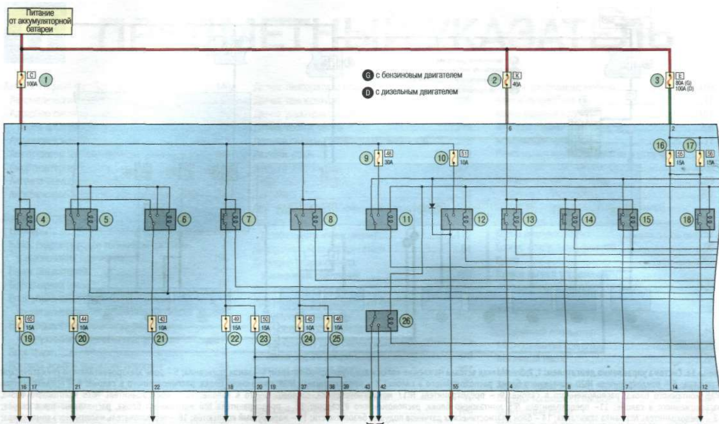
Схема 2а. Монтажные блоки, расположенные в моторном отсеке: 1 – плавкая вставка 100 А на клемме «плюс» аккумуляторной батареи; 2 – плавкая вставка 40 А на клемме «плюс» аккумуляторной батареи; 3 – плавкая вставка на клемме «плюс» аккумуляторной батареи; 4 – реле противотуманных фар; 5 – реле дальнего света (левая блок-фара); 6 – реле дальнего света (правая блок-фара); 7 – реле ближнего света; 8 – реле заднего фонаря; 9 – предохранитель №8 основного монтажного блока, расположенного в моторном отсеке; 10 – предохранитель №11 основного монтажного блока, расположенного в моторном отсеке; 11 – реле моторедуктора очистителя ветрового окна; 12 – реле компрессора кондиционера; 13 – реле 1 электровентиляторов системы охлаждения; 14 – реле 2 электровентиляторов системы охлаждения; 15 – реле 3 электровентиляторов системы охлаждения; 16 – предохранитель №15 основного монтажного блока, расположенного в моторном отсеке; 17 – предохранитель №16 основного монтажного блока, расположенного в моторном отсеке; 18 – реле обогрева окна двери задка; 19 – предохранитель №25 основного монтажного блока, расположенного в моторном отсеке; 20 – предохранитель №4 основного монтажного блока, расположенного в моторном отсеке; 21 – предохранитель №3 основного монтажного блока, расположенного в моторном отсеке; 22 – предохранитель №10 основного монтажного блока, расположенного в моторном отсеке; 23 – предохранитель №9 основного монтажного блока, расположенного в моторном отсеке; 24 – предохранитель №25 основного монтажного блока, расположенного в моторном отсеке; 25 – предохранитель №5 основного монтажного блока, расположенного в моторном отсеке; 26 – реле моторедуктора очистителя окна двери задка
