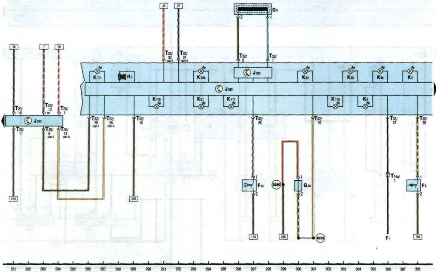
Схема 7л. Базовая комплектация автомобиля с двигателем 1,6 л (75 кВт)
