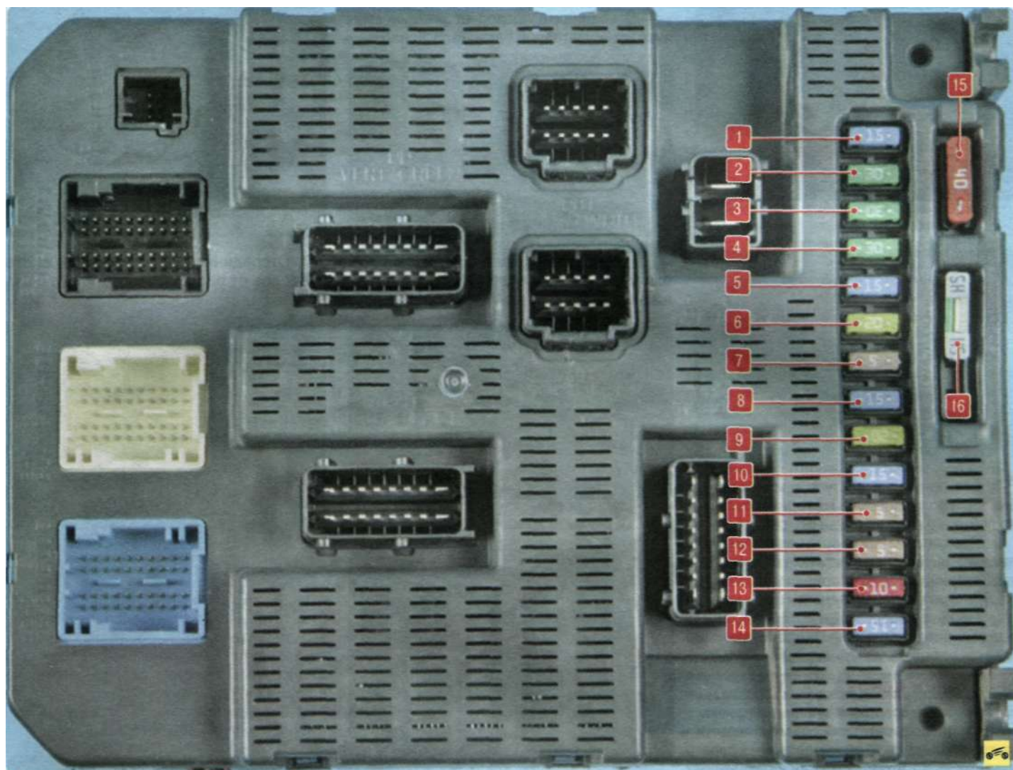
Рис. 10.3. Монтажный блок, расположенный в салоне автомобиля
