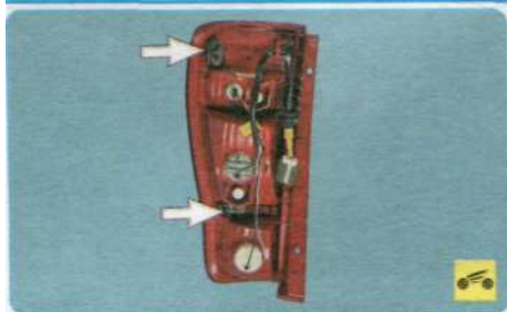
Так расположены фиксаторы заднего фонаря
