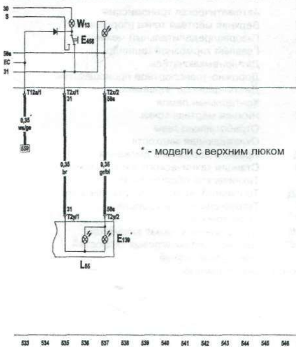
32 Переключатель управления верхним люком, передний пассажирский светильник для чтения и его выключатель
