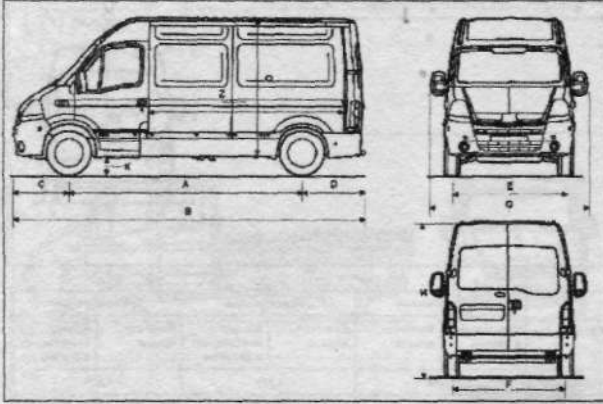
Габаритные размеры, м
