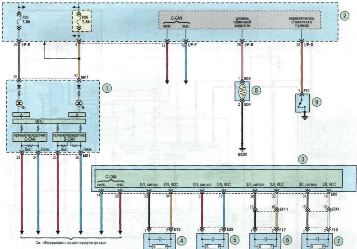
Схема 4в. Антиблокировочная система тормозов: 1 – панель приборов; 2 – блок предохранителей в салоне автомобиля; 3 – блок управления ABS; 4 – датчик левого переднего колеса; 5 – датчик правого переднего колеса; 6 – датчик левого заднего колеса; 7 – датчик правого заднего колеса; 8 – датчик уровня тормозной жидкости; 9 – переключатель стояночного тормоза
