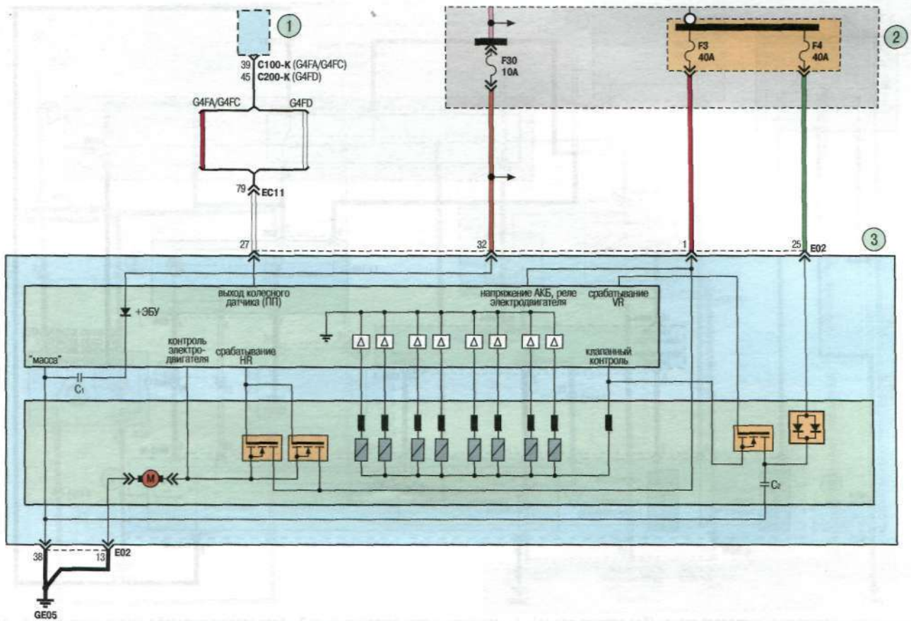
Схема 4б. Антиблокировочная система тормозов: 1 – блок управления двигателем; 2 – блок предохранителей в моторном отсеке; 3 – блок управления ABS
