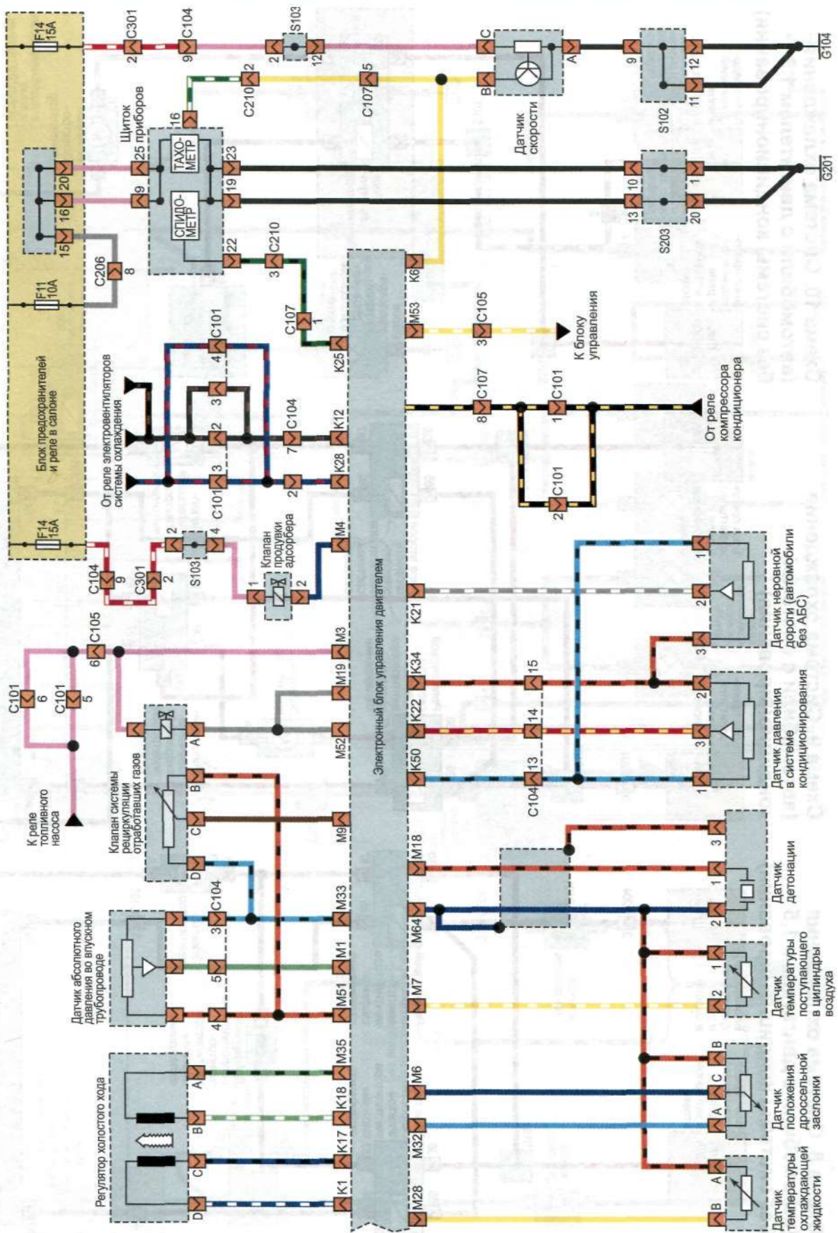
Схема 7. Система управления двигателем 1,5 (ОКОНЧАНИЕ)
