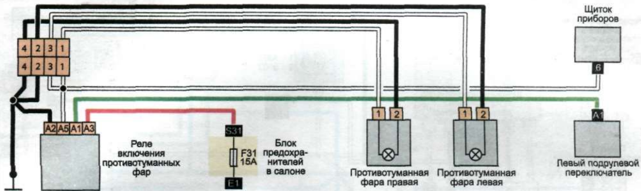
Схема 11. Противотуманные фары
