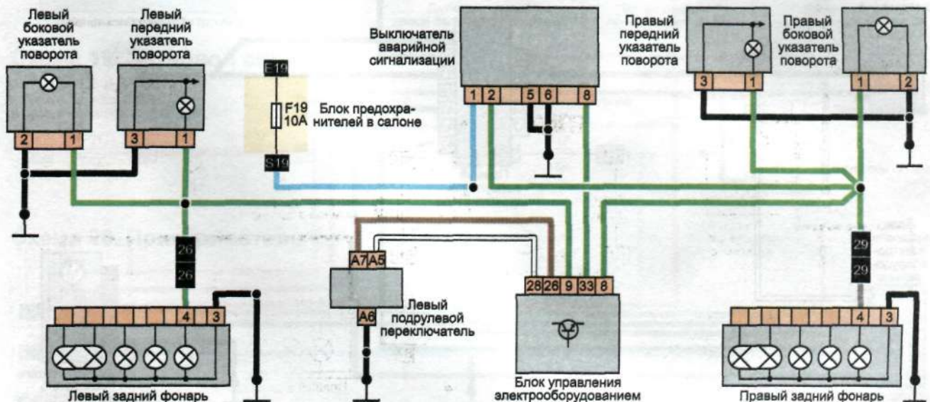
Схема 14 Указатели поворота и аварийная сигнализация
