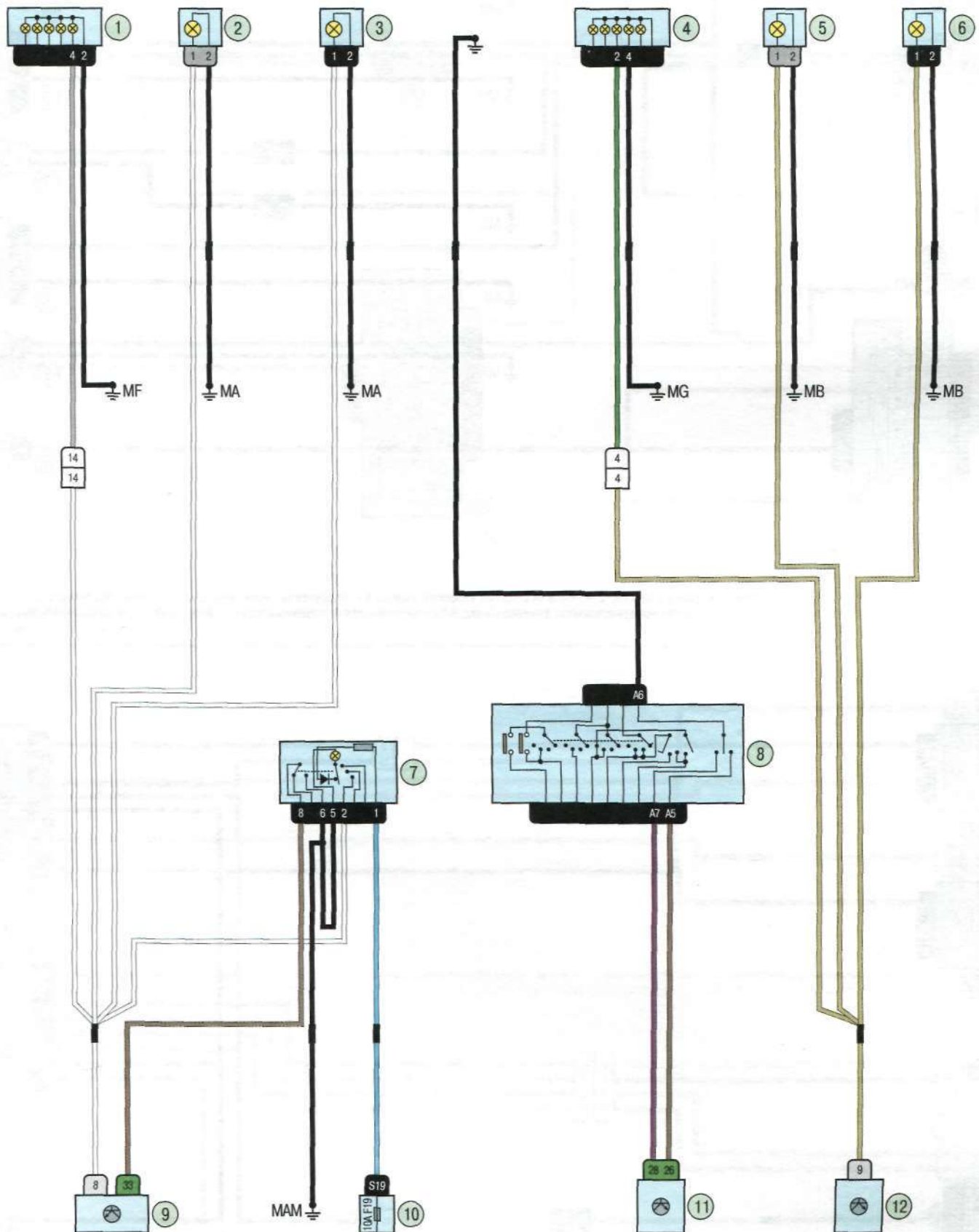
Схема 11. Указатели поворота и аварийная сигнализация: 1 – правый задний фонарь; 2 – лампа правого переднего указателя поворота; 3 – правый боковой указатель поворота; 4 – левый задний фонарь; 5 – лампа левого переднего указателя поворота; 6 – правый боковой указатель поворота; 7 – выключатель аварийной сигнализации; 8 – подрулевой переключатель; 9, 11, 12 – блок управления электрооборудованием салона; 10 – блок предохранителей в салоне
