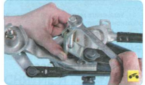
7. Отверните гайку крепления кривошипа.
