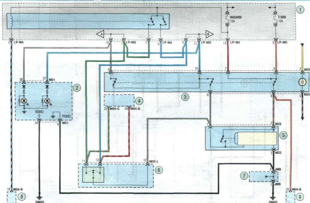
Схема 19а. Лампы указателей поворота и аварийной сигнализации: 1 – монтажный блок в салоне; 2 – комбинация приборов; 3 – выключатель аварийной сигнализации; 4, 8, 9 – блок управления электрооборудованием кузова; 5 – прерыватель указателей поворота; 6 – подрулевой переключатель наружного освещения и указателей поворота; 7 – соединительный разъем
