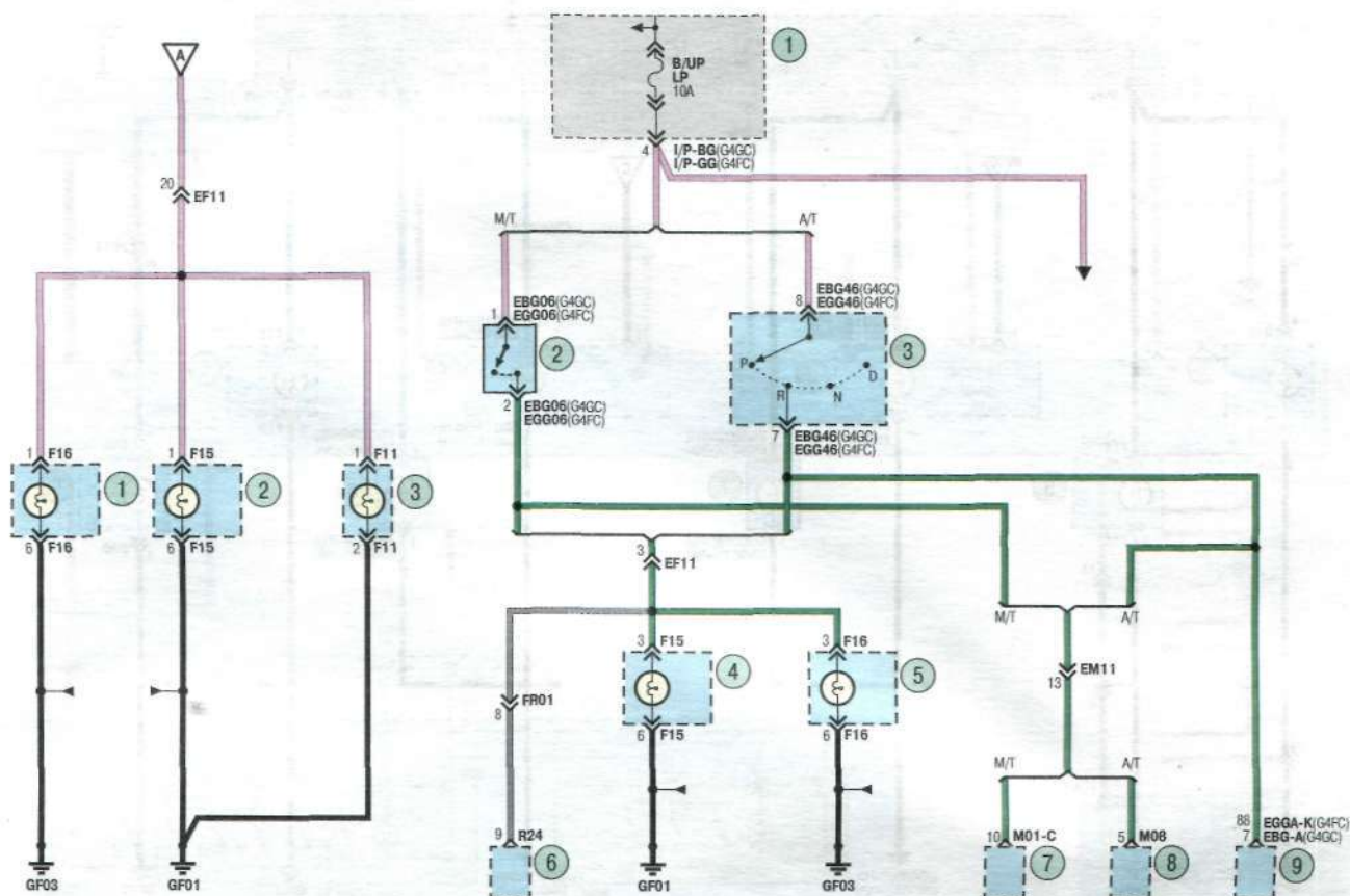
Схема 176. Лампы стоп-сигнала: 1 – лампа стоп-сигнала/заднего габаритного огня правого заднего фонаря; 2 – лампа стоп-сигнала/заднего габаритного огня левого заднего фонаря; 3 – лампы дополнительного стоп-сигнала
