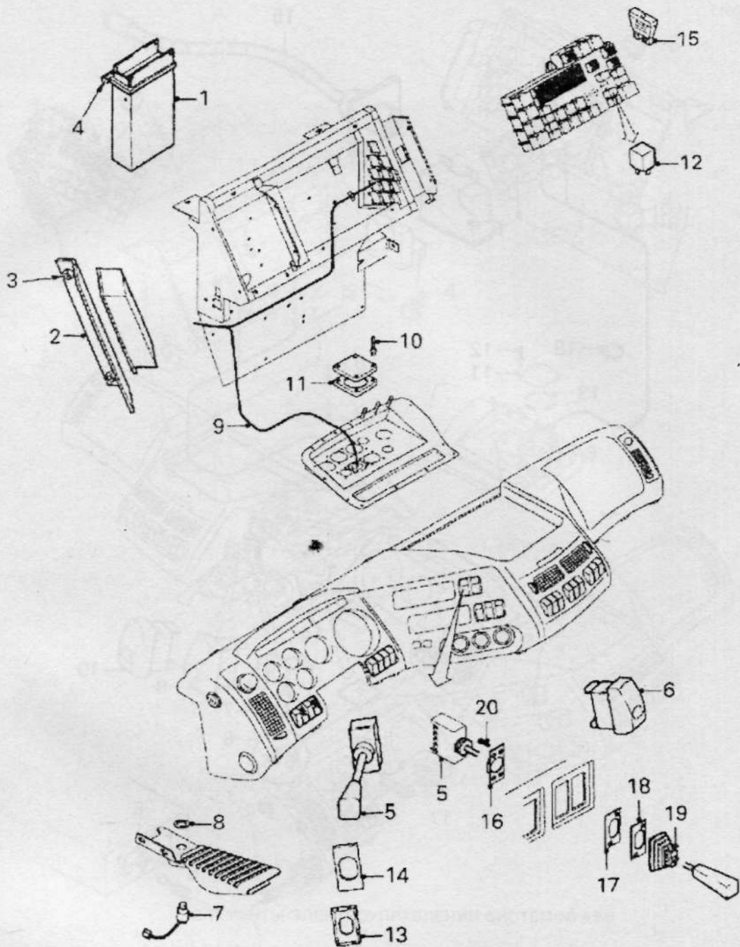
ЭЛЕМЕНТЫ ЭЛЕКТРОУПРАВЛЕНИЯ РЕТАРДЕРОМ
