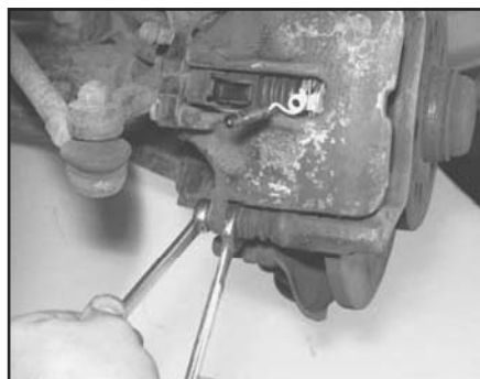
Рис. 4.4. Отверните и извлеките болт нижнего направляющего пальца суппорта, удерживая палец от проворота гаечным ключом
