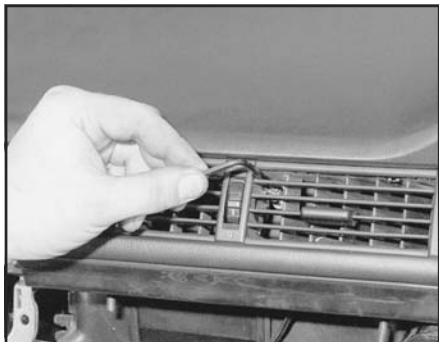
Рис. 30.14,а. Выверните винт из соединительного звена заслонки приточного воздуха
