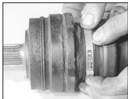
Рис. 6.17,а. Натяните и зафиксируйте хомут на чехле
