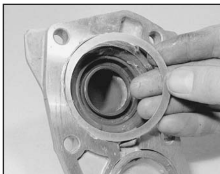
Рис. 4.4. Снимите дистанционное кольцо(а)
