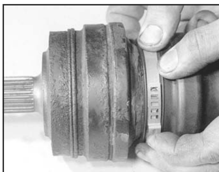
Рис. 6.17,б. Выберите слабину хомута, сжимая его выступ
