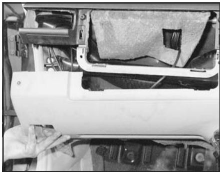
Рис. 30.12,б. Выверните винты и снимите нижнюю лицевую панель со стороны водителя
