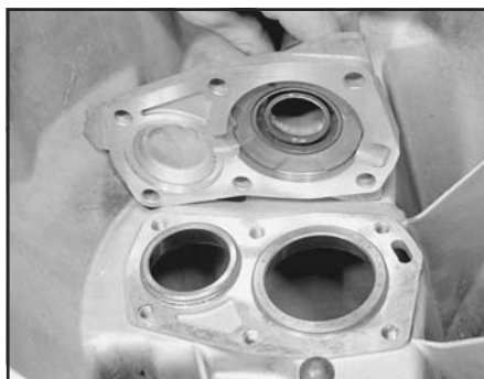
Рис. 4.3. Снятие крышки коробки передач
