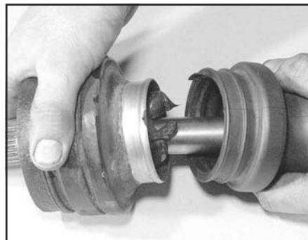
Рис. 6.16,а. Установите новый чехол
