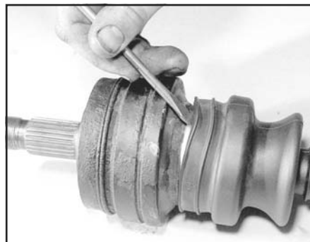
Рис. 6.16,б. Приподнимите наружную уплотнительную кромку чехла для выравнивания внутри него давления воздуха
