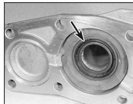
Рис. 4.5. Расположение манжеты (показана стрелкой) входного вала
