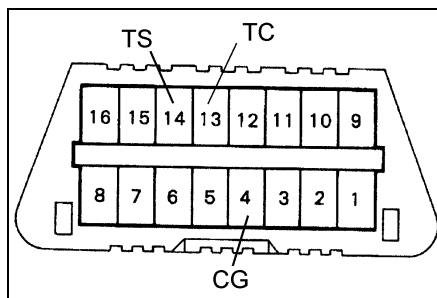
Разъем DLC3 (с 07.2000 г.).
