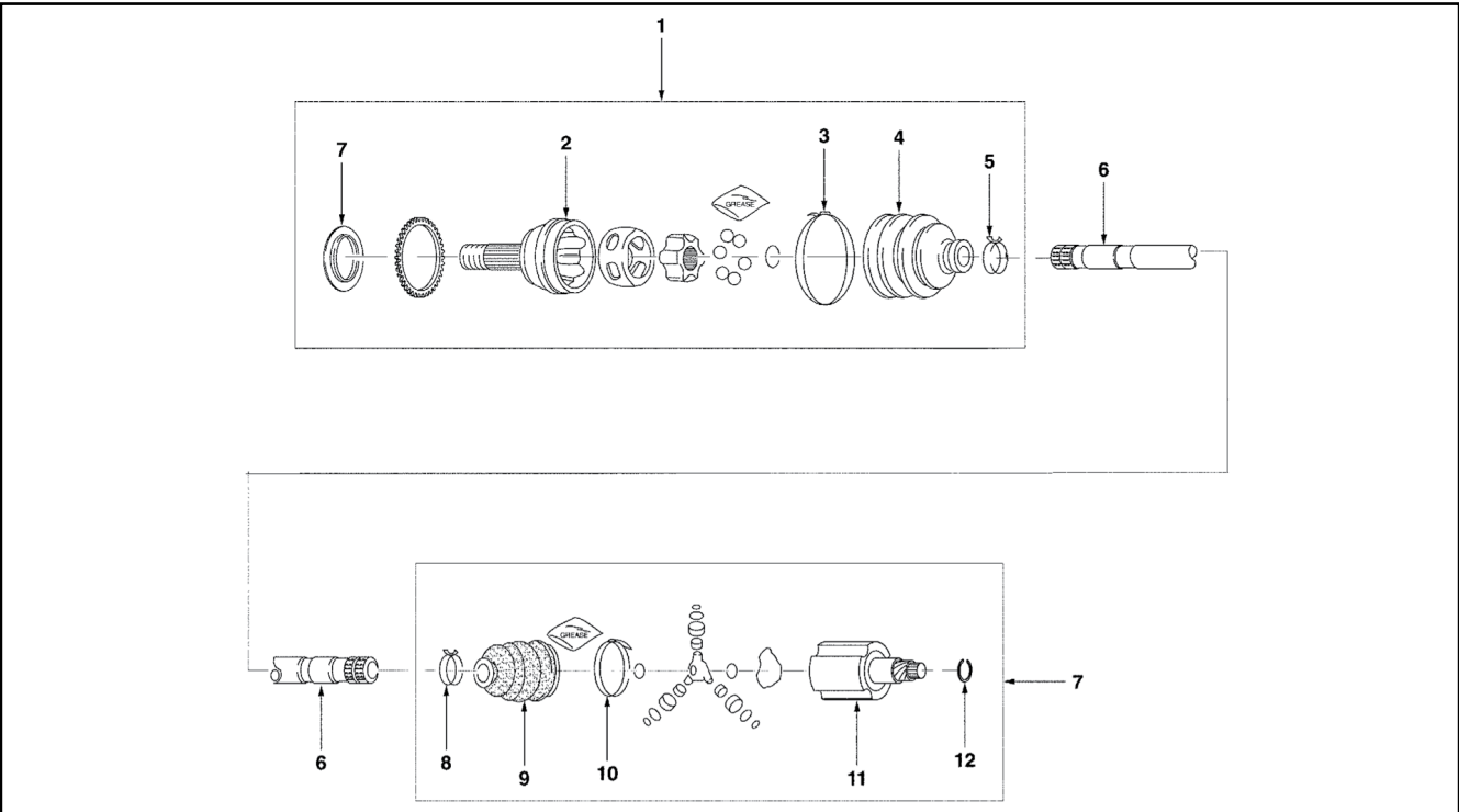
Передний мост в сборе: 1. Наружное шарнирное соединение в сборе; 2. Наружный шарнир; 3. Хомут для крепления защитного кожуха; 4. Внешний защитный кожух полуоси; 5. Хомут для крепления защитного кожуха; 6. Полуось привода колеса (показана левая полуось; правая полуось аналогична); 7. Внутреннее шарнирное соединение в сборе; 8. Хомут для крепления защитного кожуха; 9. Внутренний защитный кожух полуоси; 10. Хомут для крепления защитного кожуха; 11. Корпус внутреннего шарнира; 12. Упорное кольцо
