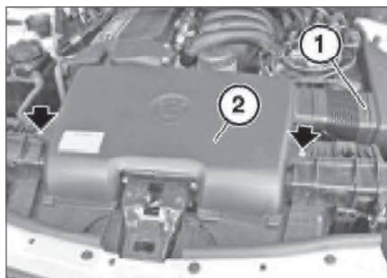
Рис. 5.31. Впускной канал
