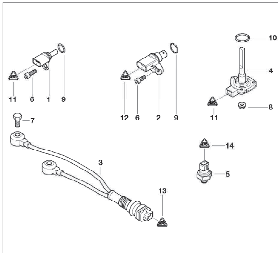
Рис. 10.7. Датчики системы управления:
