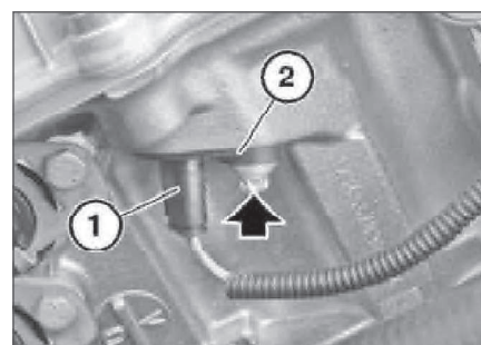
Рис. 10.9. Датчик впускного распределительного вала
