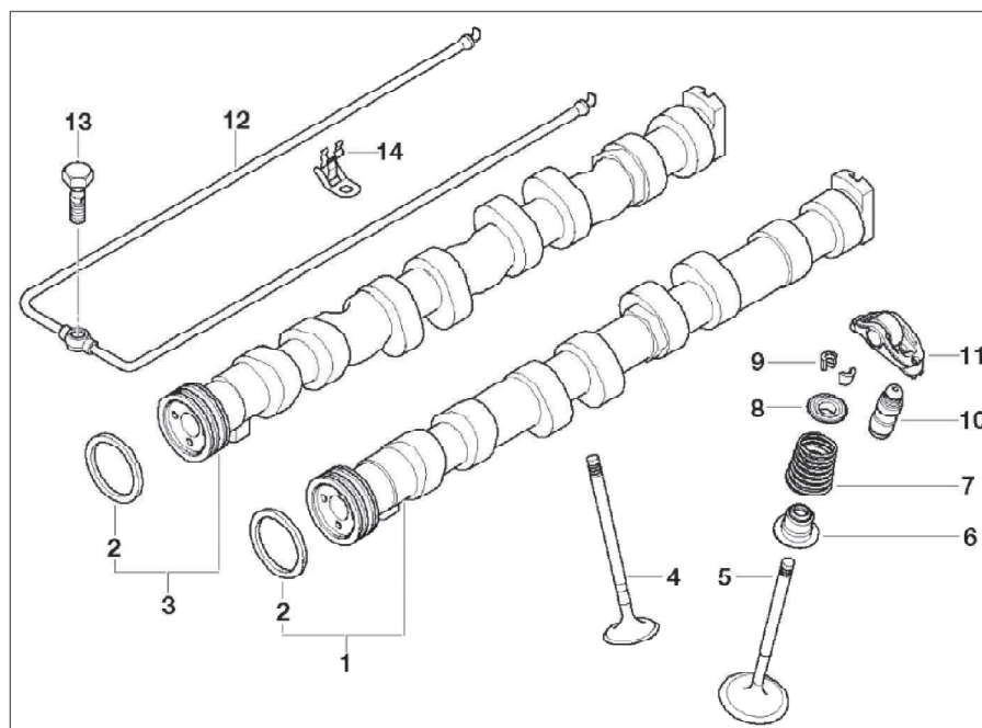
Рис. 3.176. Распределительные валы:
