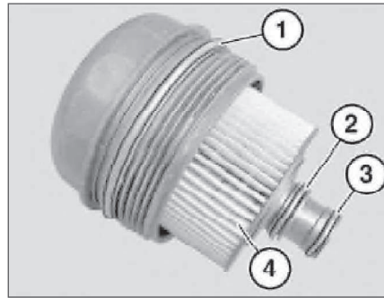
Рис. 2.10. Кольца фильтра
