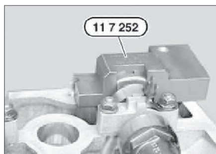
Рис. 3.174. Приспособление «11.7.252»
