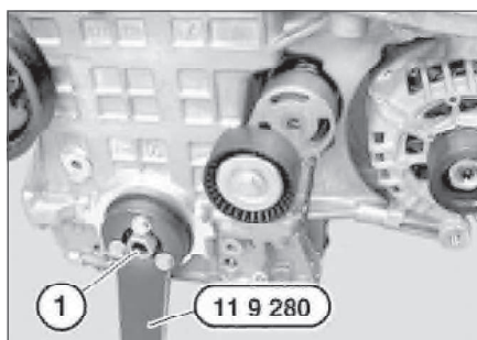
Рис. 4.42. Планка цепи
