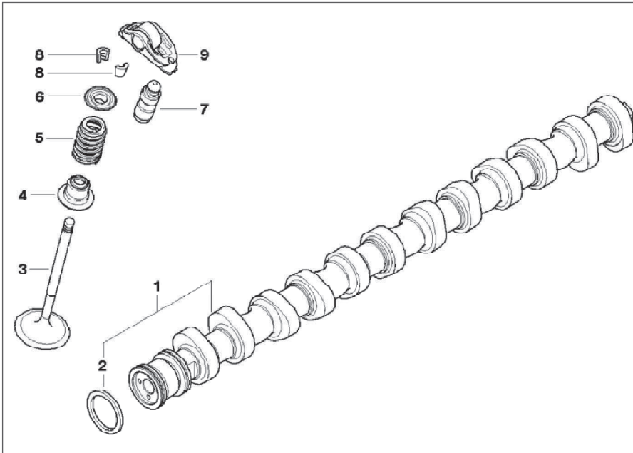
Рис. 7.120. Клапанный механизм:
