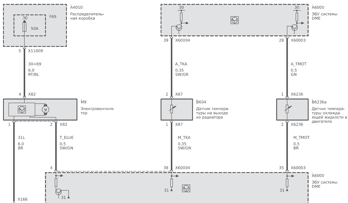
Рис. 11.20. Система охлаждения двигателя (N52—MSV70)
