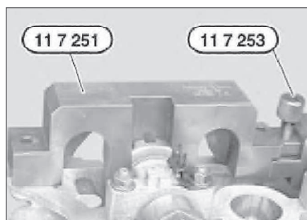
Рис. 3.175. Приспособление «11.7.251»
