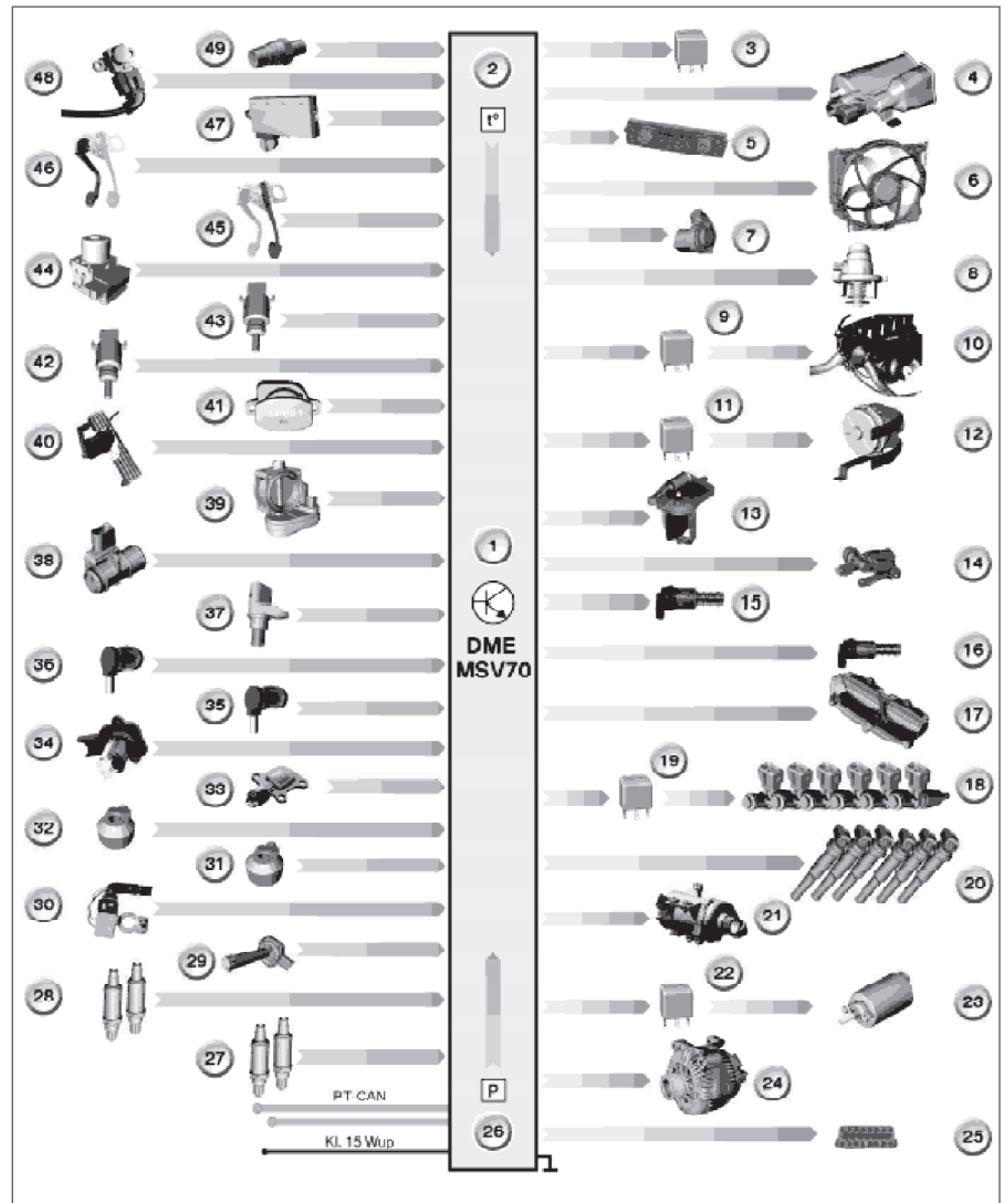
Рис. 6.37. Датчики системы управления:
