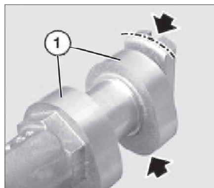
Рис. 3.177. Лыска вала
