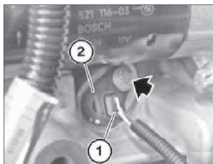
Рис. 10.8. Датчик коленвала
