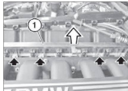
Рис. 6.224. Магистраль
