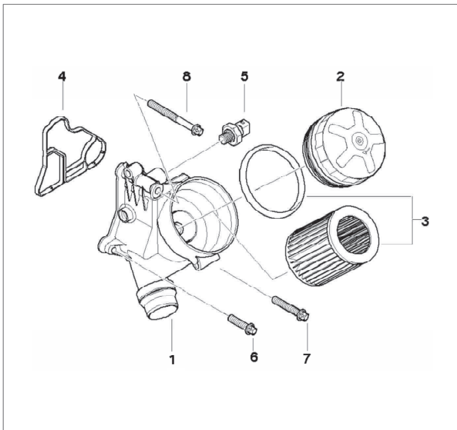
Рис. 6.220. Масляный фильтр.
