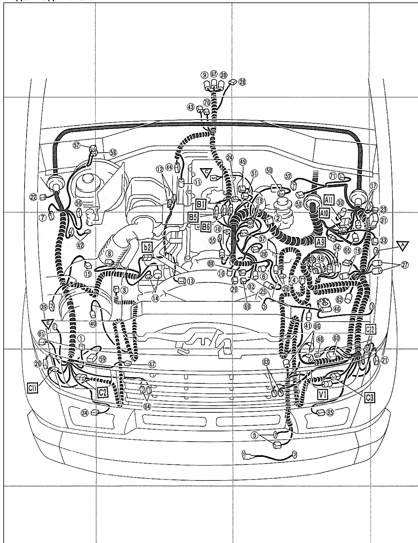
Моторный отсек.
